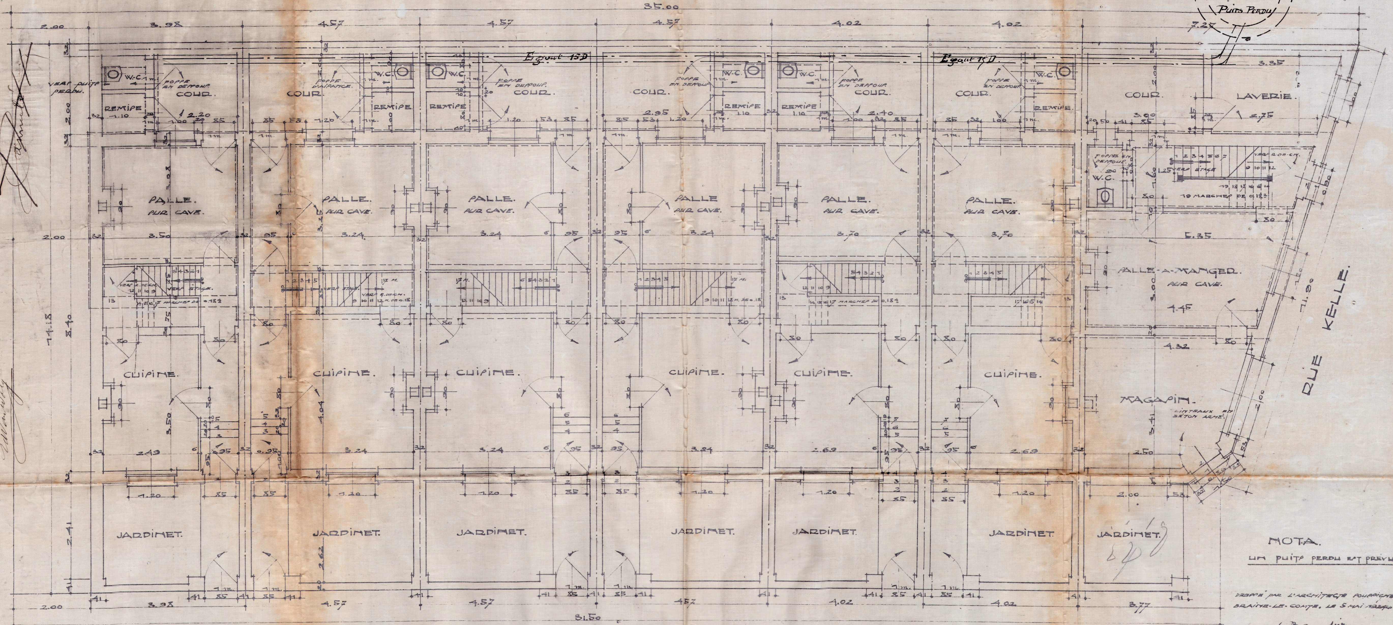
PLAN DU REZ-DE-CHAUSSEE.
