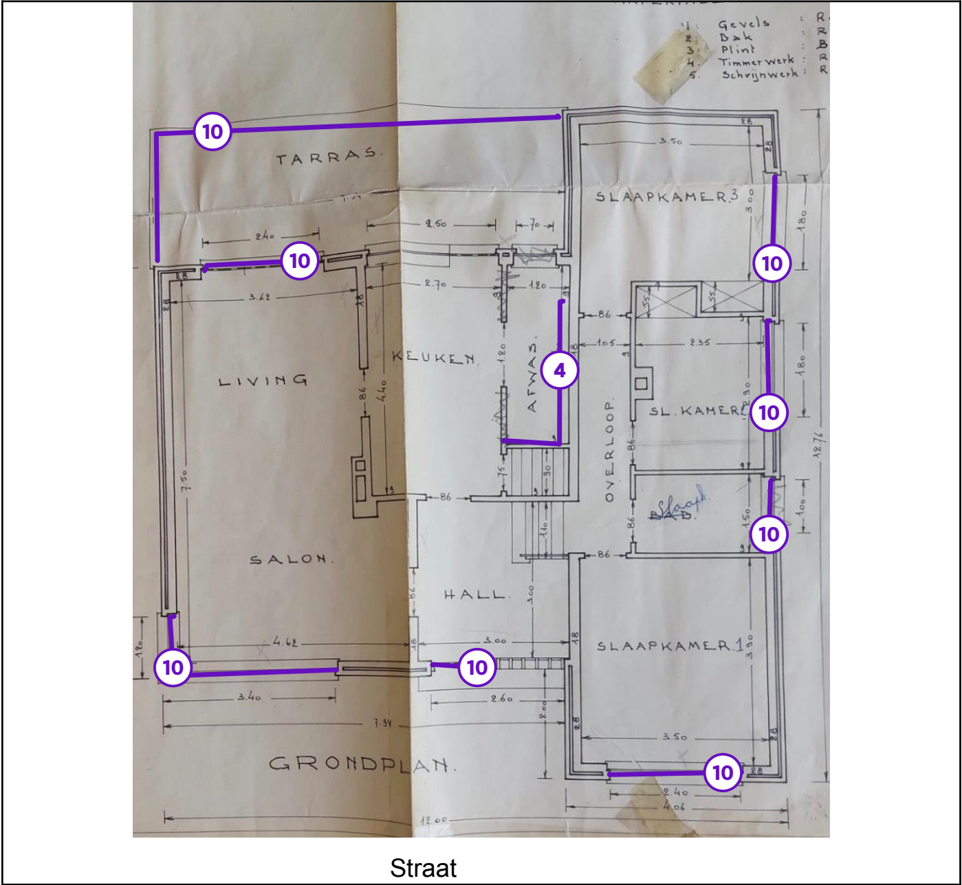
Legende van plan 1.4: Gelijkvloers kopie
