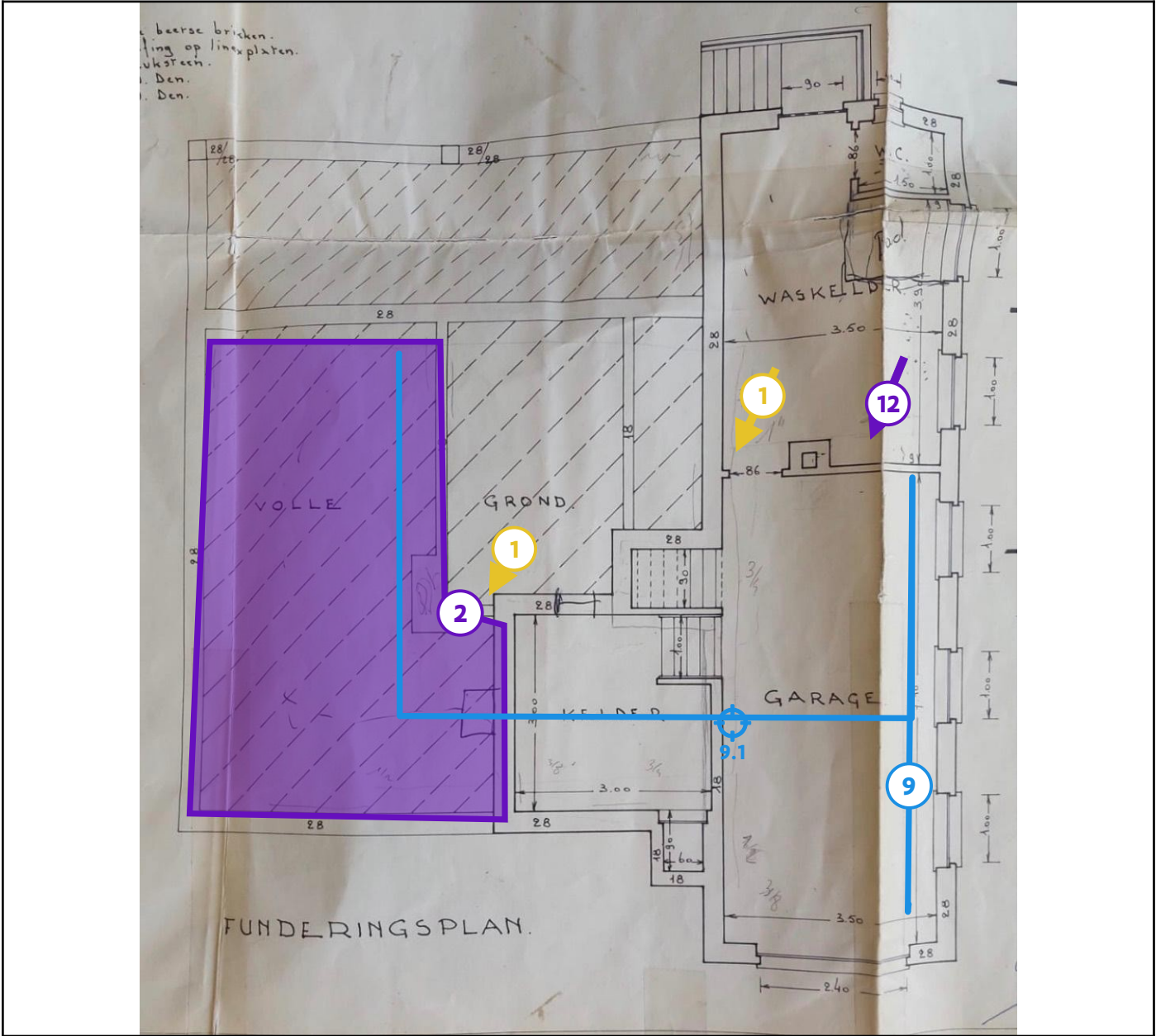
Legende van plan 1.5: Kelder
