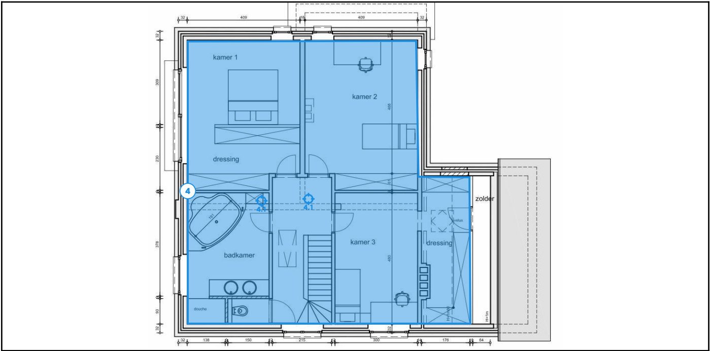
Legende van plan 1.11: Eertse verdieping plan - pleister plafonds
