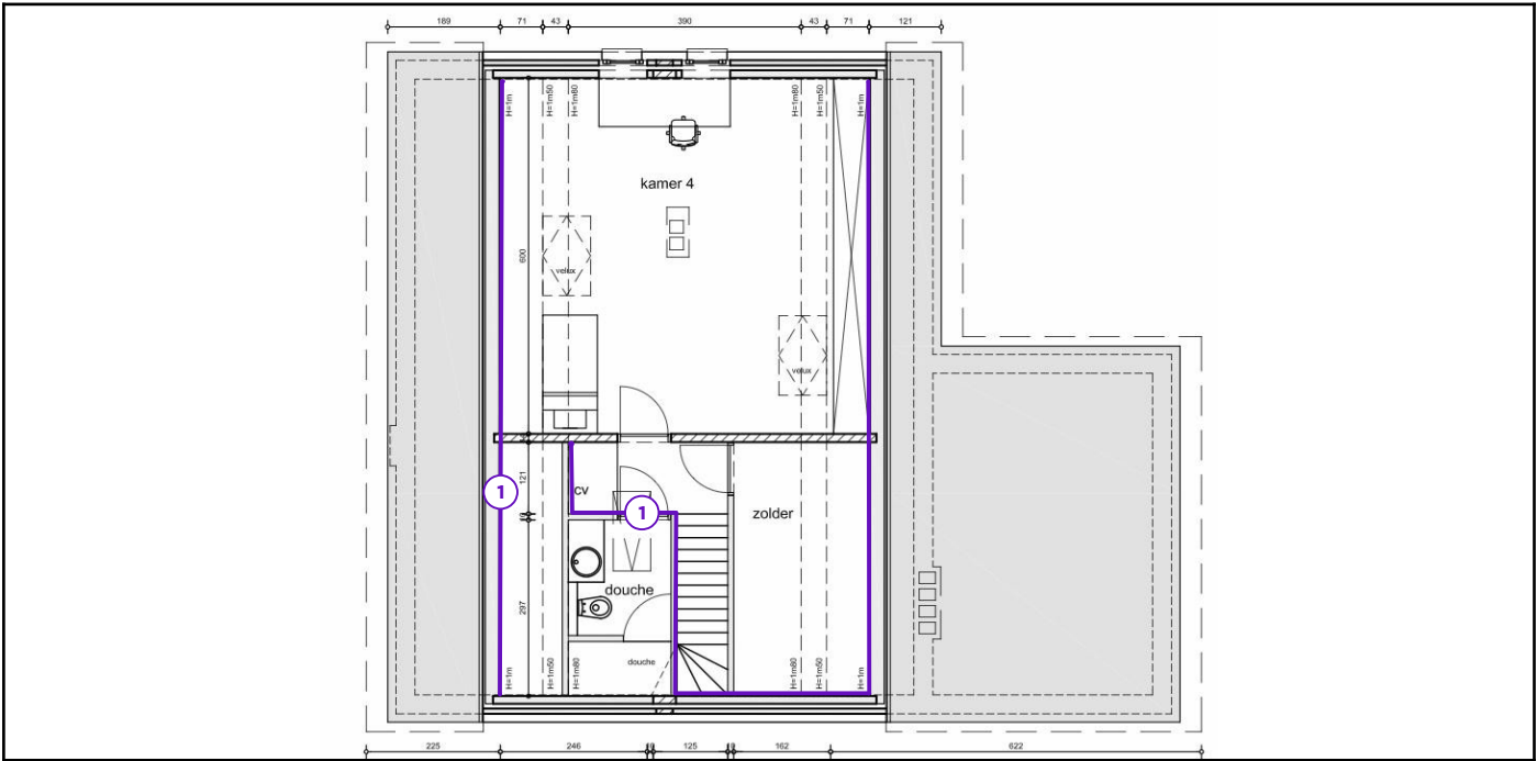
Legende van plan 1.9: Zolder plan - voorzetwanden
