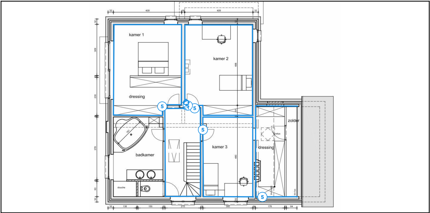
Legende van plan 1.7: Eertse verdieping plan - pleister muren
