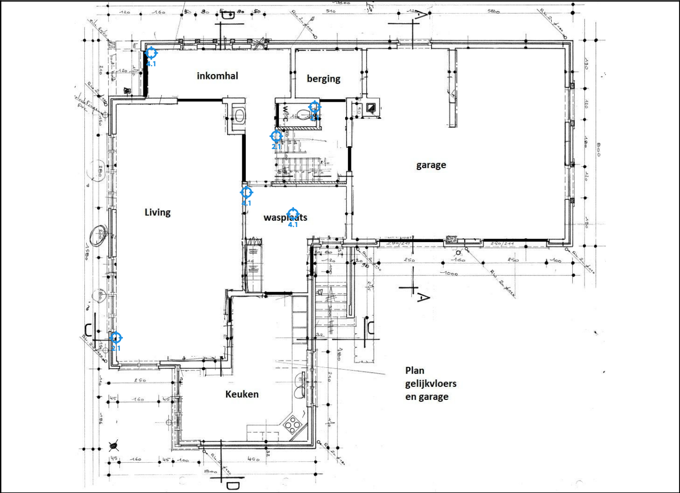
Legende van plan 1.1: plan gelijkvloers en garage
