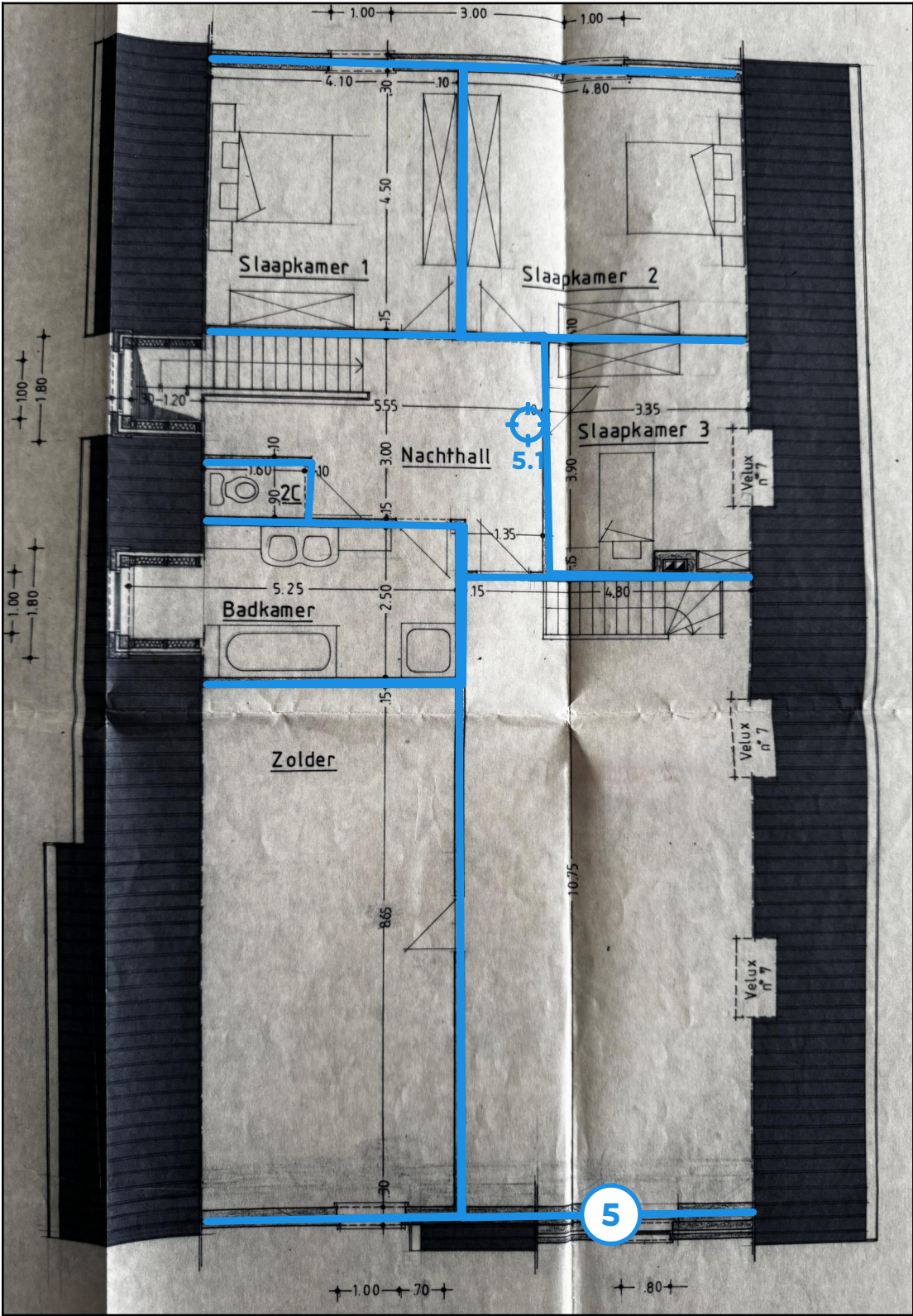
Legende van plan 1.4: Verdieping V+1
