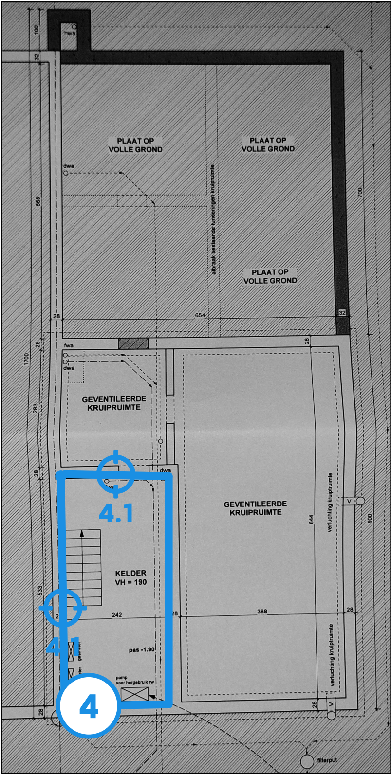
Legende van plan 1.1: Kelder
