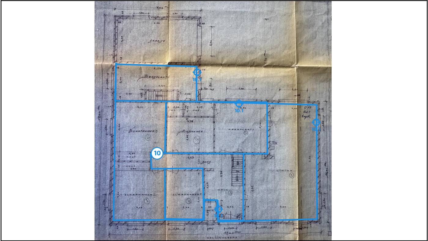
Legende van plan 1.4: Woning - Gelijkvloers (wand)
