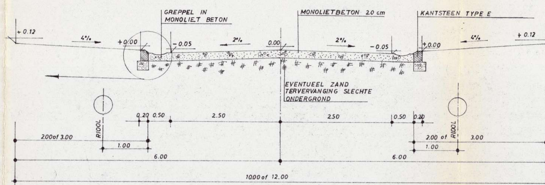
MODELWARSPROFIEL BETONWEG schaal 1/50
