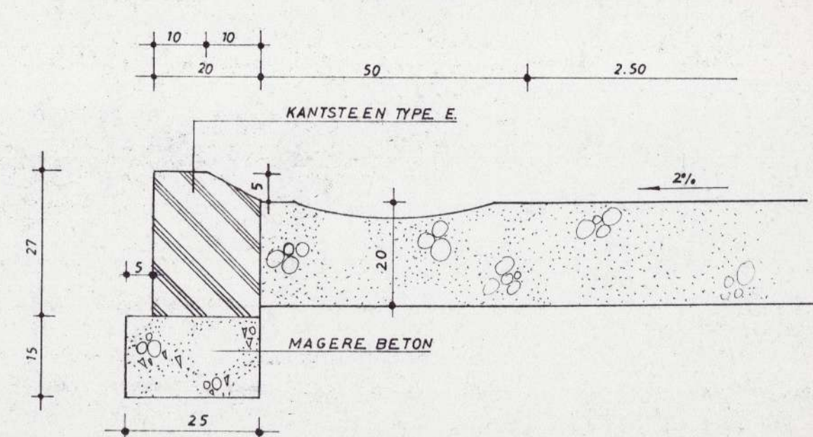
DEELTEKENING schaal: 1/10
