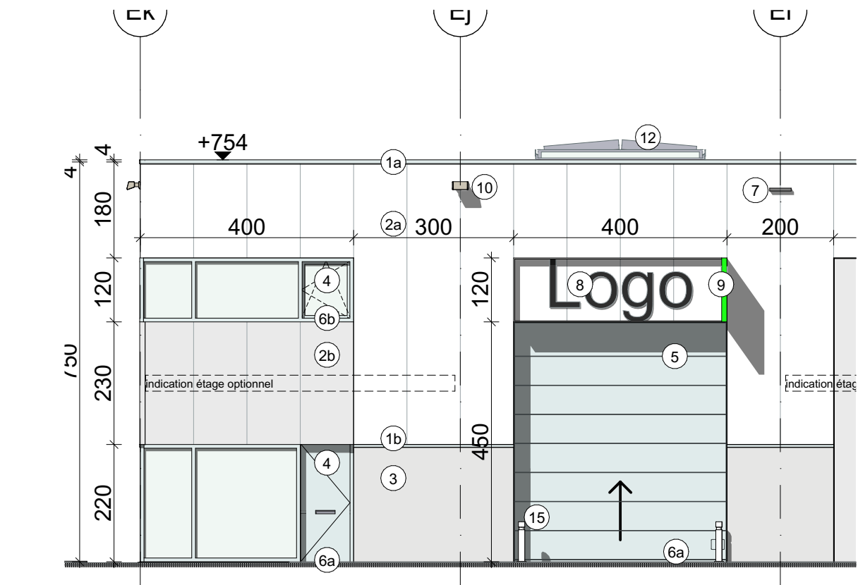
façade arrière
