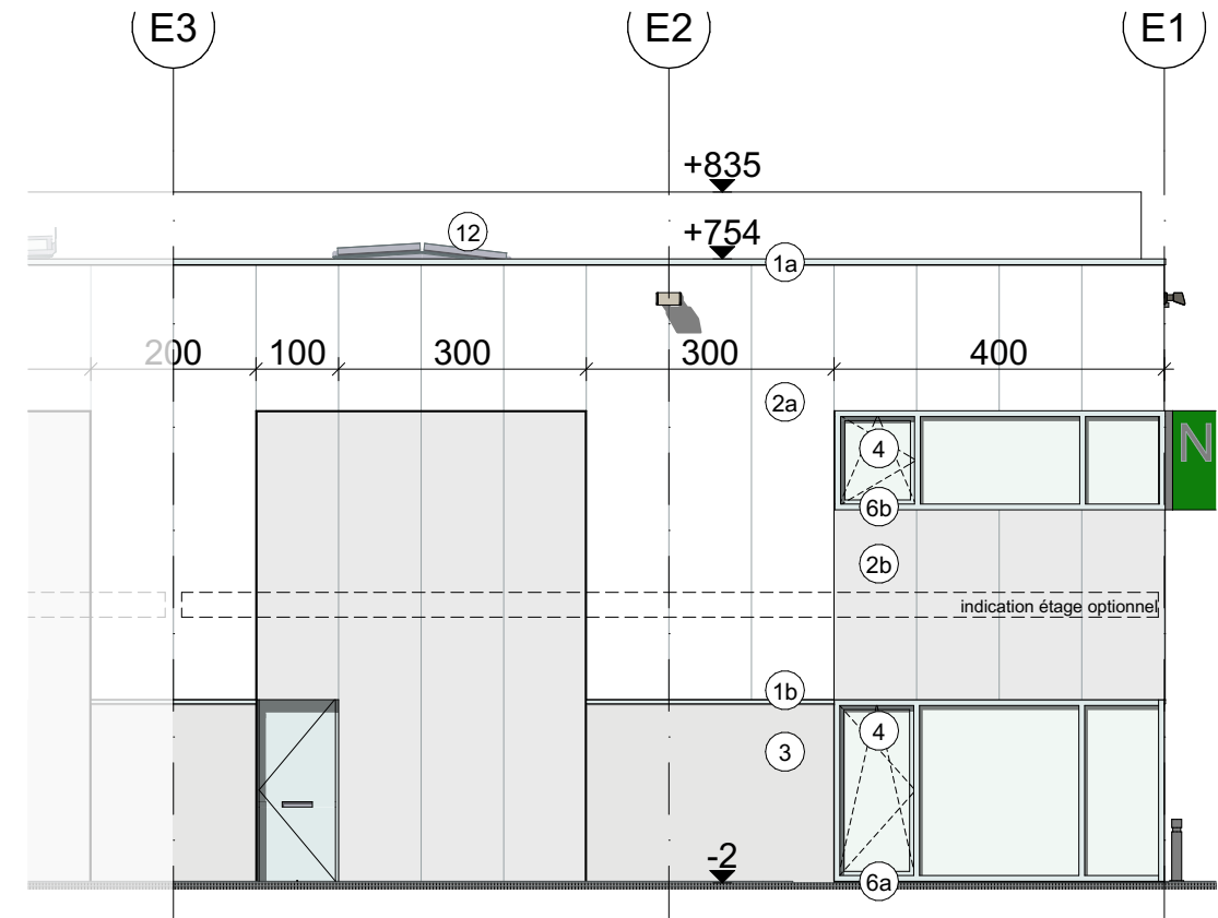
façade droite
