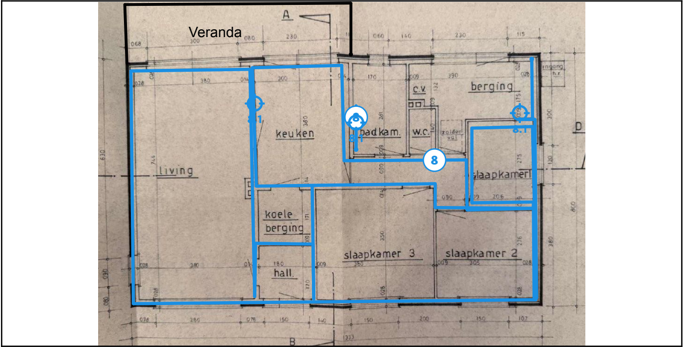
Legende van plan 1.5: Gelijkvloers
