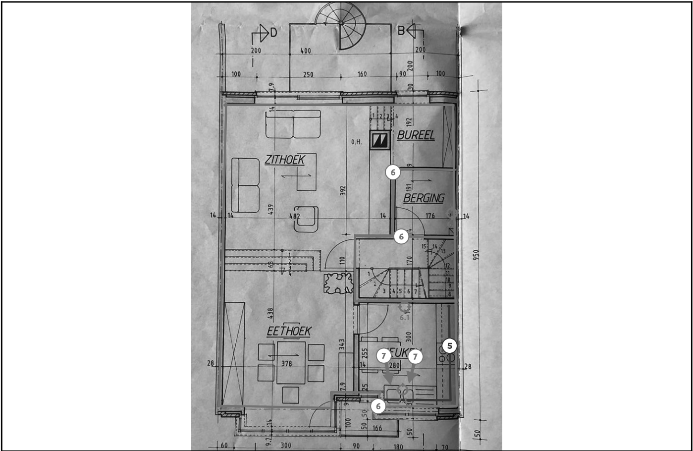
Legende van plan 1.4: Eerste Verdieping - Muren
