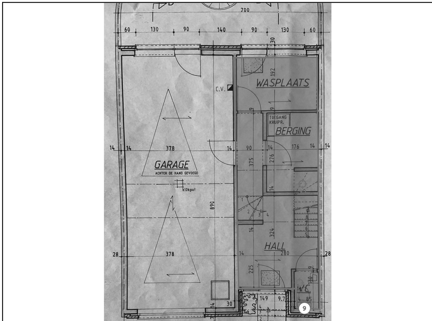
Legende van plan 1.3: Gelijkvloers - Plafonds
