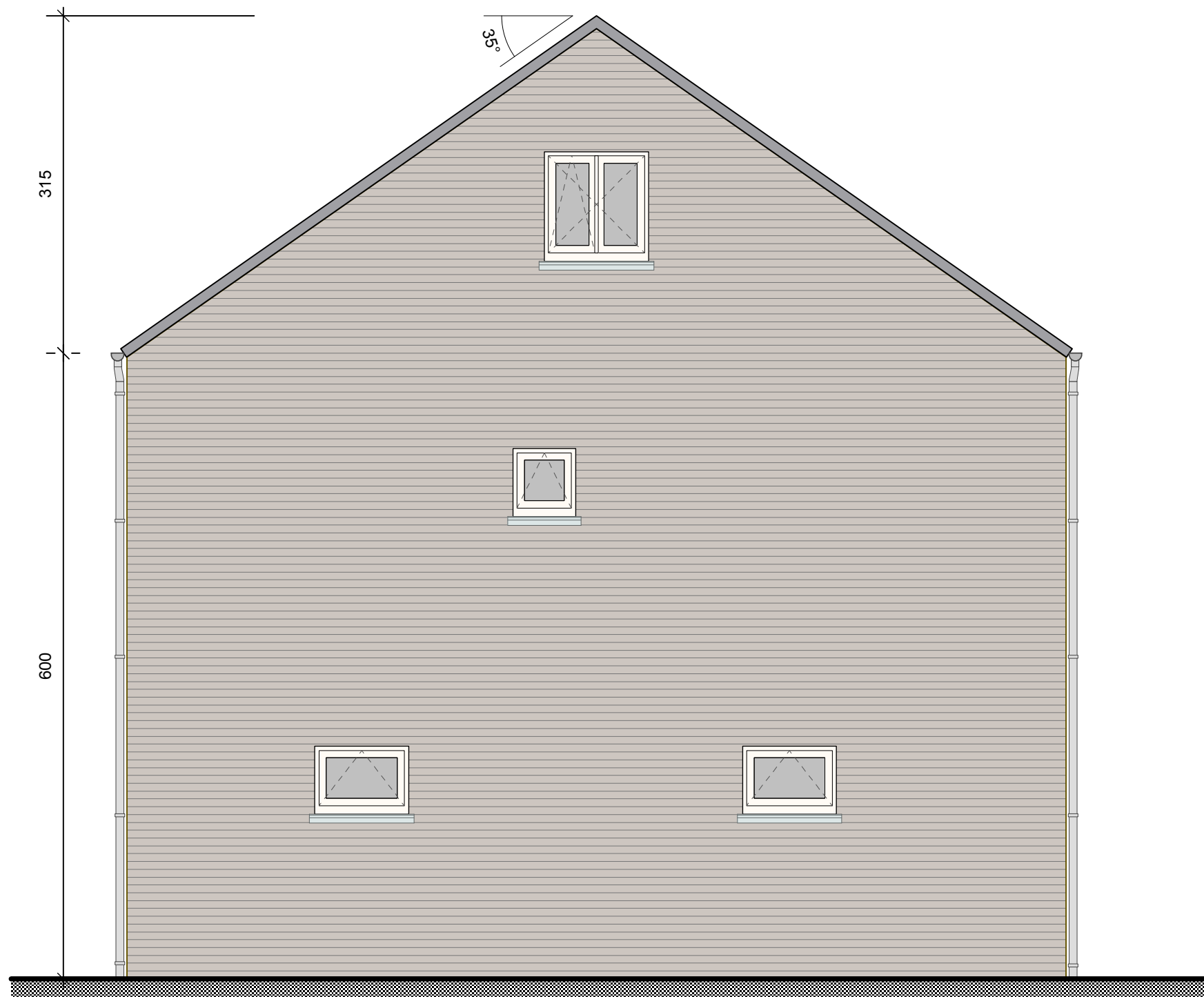
Zijgevel links
