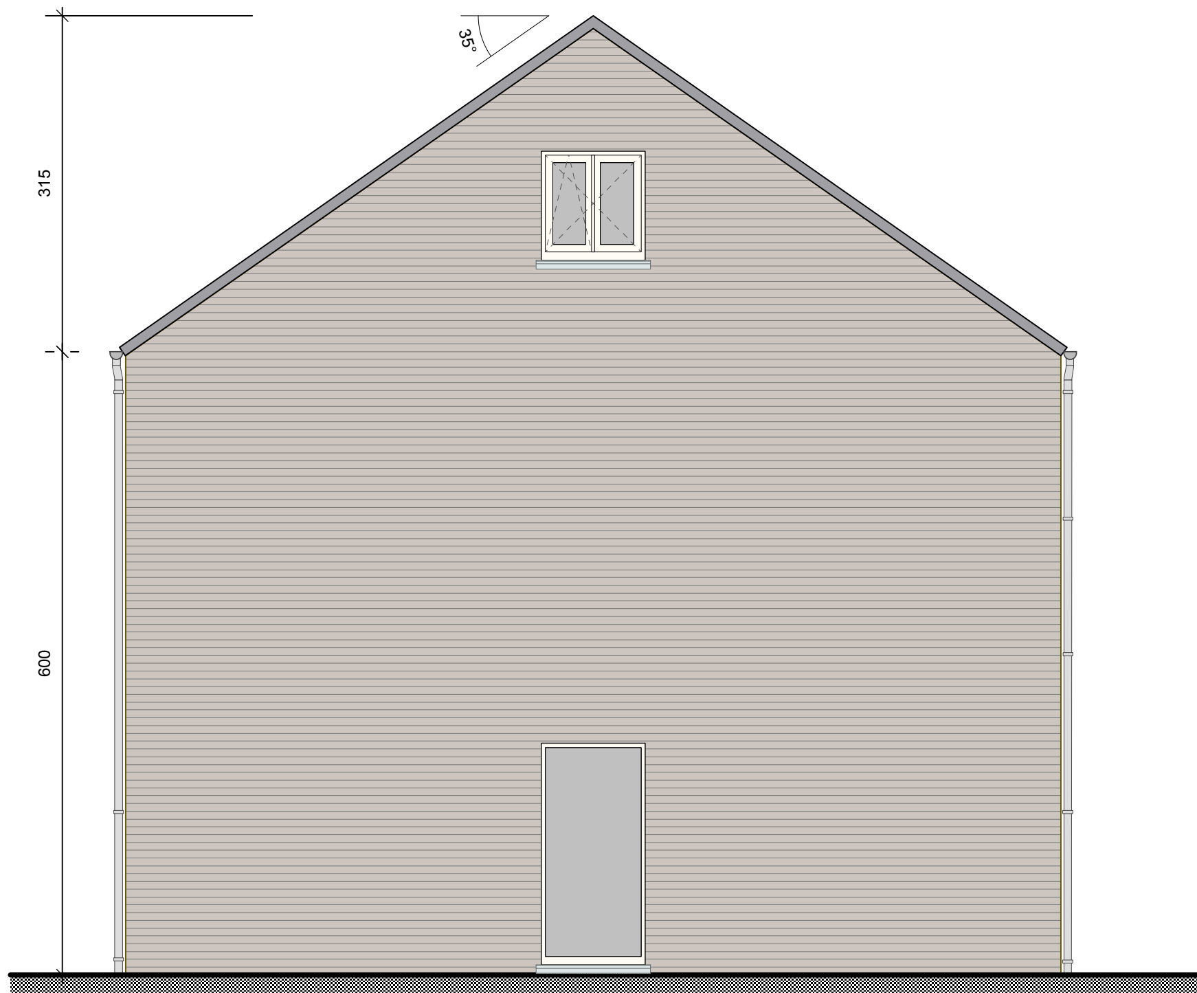
Zijgevel rechts
