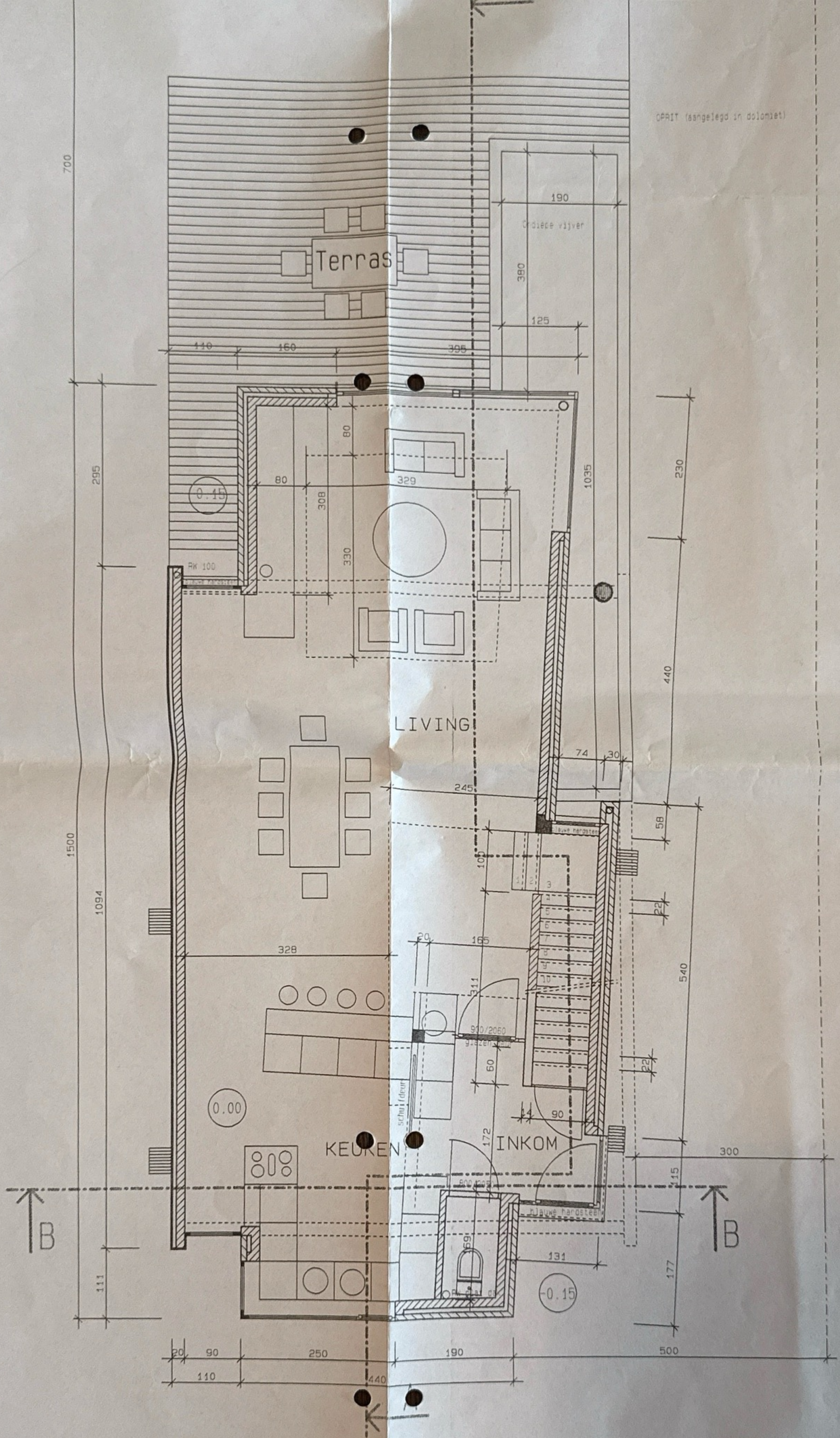
GRONDPLAN GELIJKVLOERS
