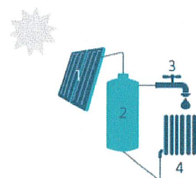
1. Zonnecollector | 2. Opslagvat zonnecollector | 3. Sanitair warm water | 4. Type element voor ruimteverwarming Optioneel
