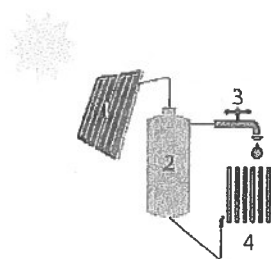
1. Zonnecollector | 2. Opslagvat zonnecollector 3. Sanitair warm water | 4. Afgeleide warmte voor ruimteverwarming verbruikt
