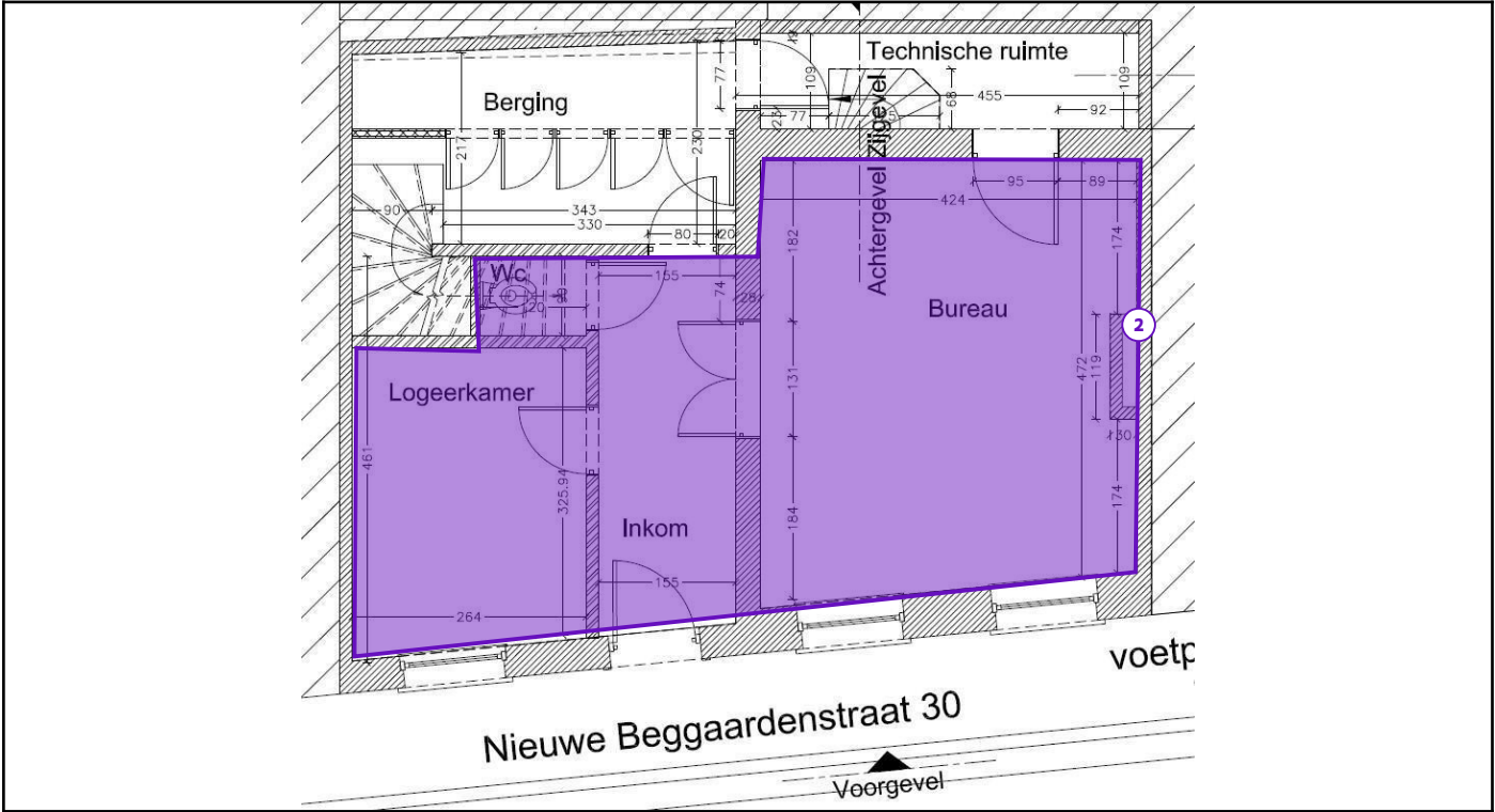
Legende van plan 1.6: GRONDPLAN NIV+0 PLAFONDS
