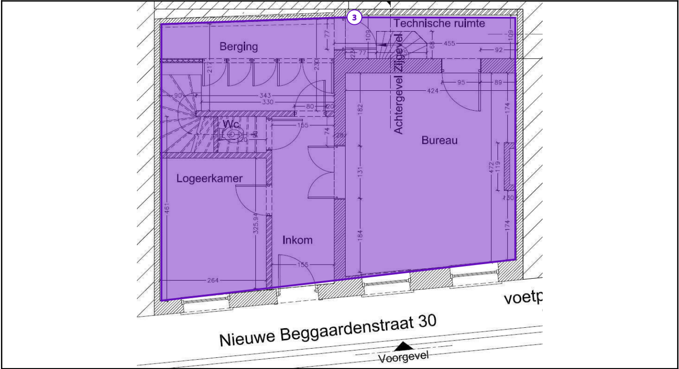
Legende van plan 1.7: GRONDPLAN NIV+0 VLOEREN
