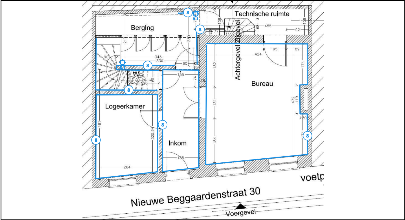
Legende van plan 1.5: GRONDPLAN NIV+0 MUREN
