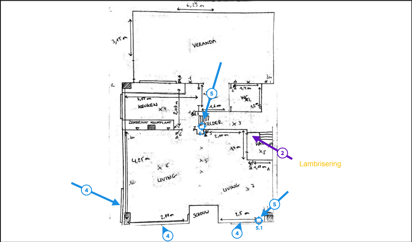
Legende van plan 1.1: schets gelijksvloer
