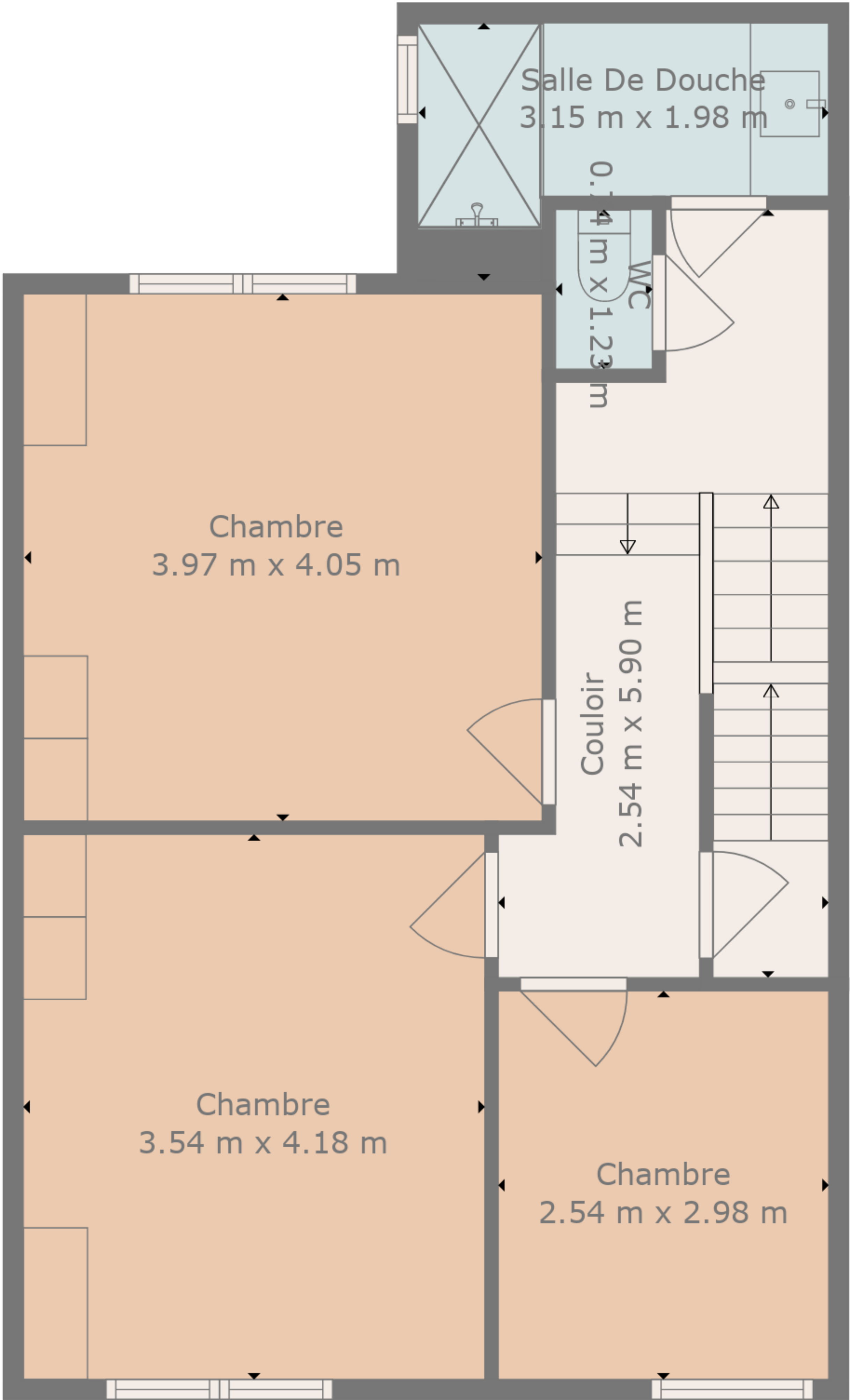
Étage 3
