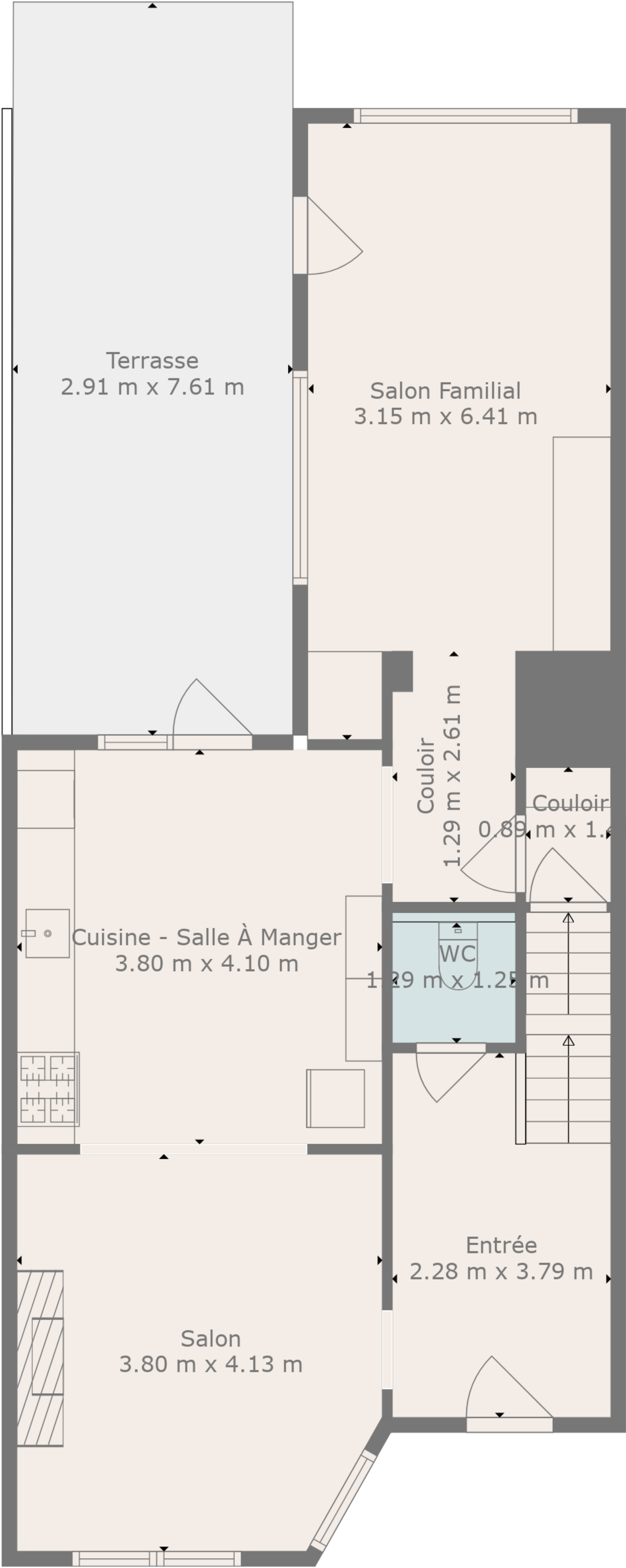
Étage 2
