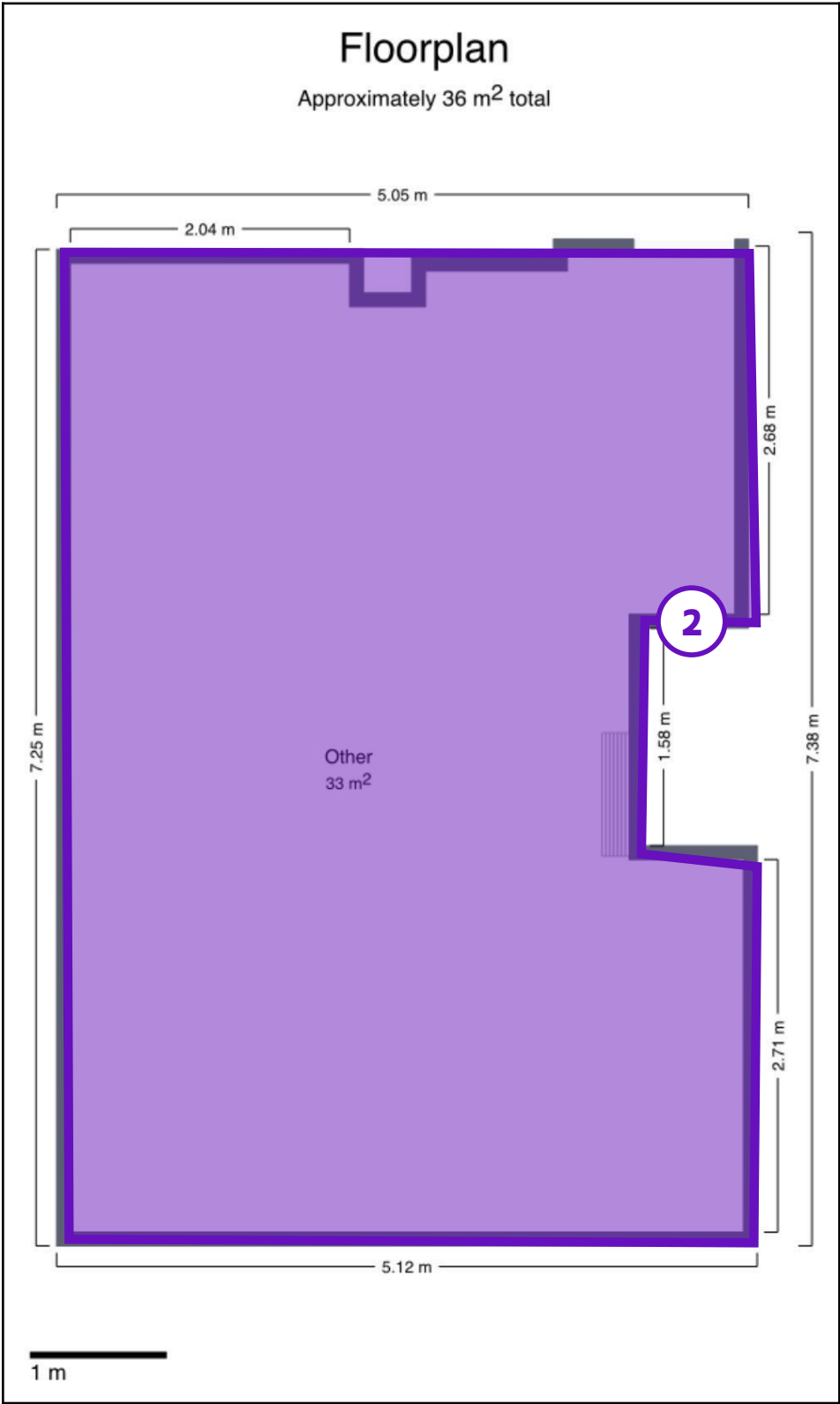
Legende van plan 1.3: Kelder kopie kopie
