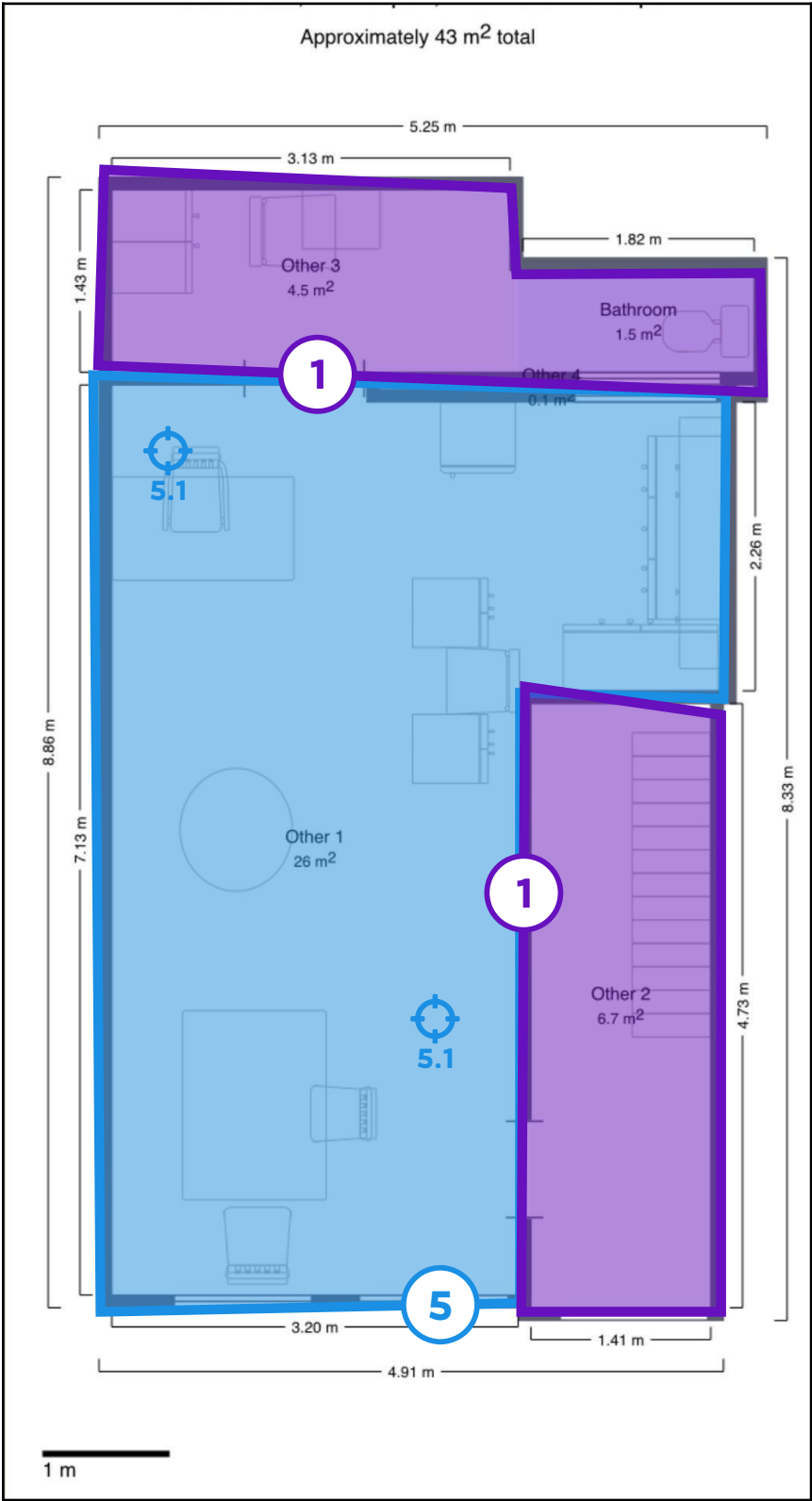
Legende van plan 1.5: Gelijkvloers kopie
