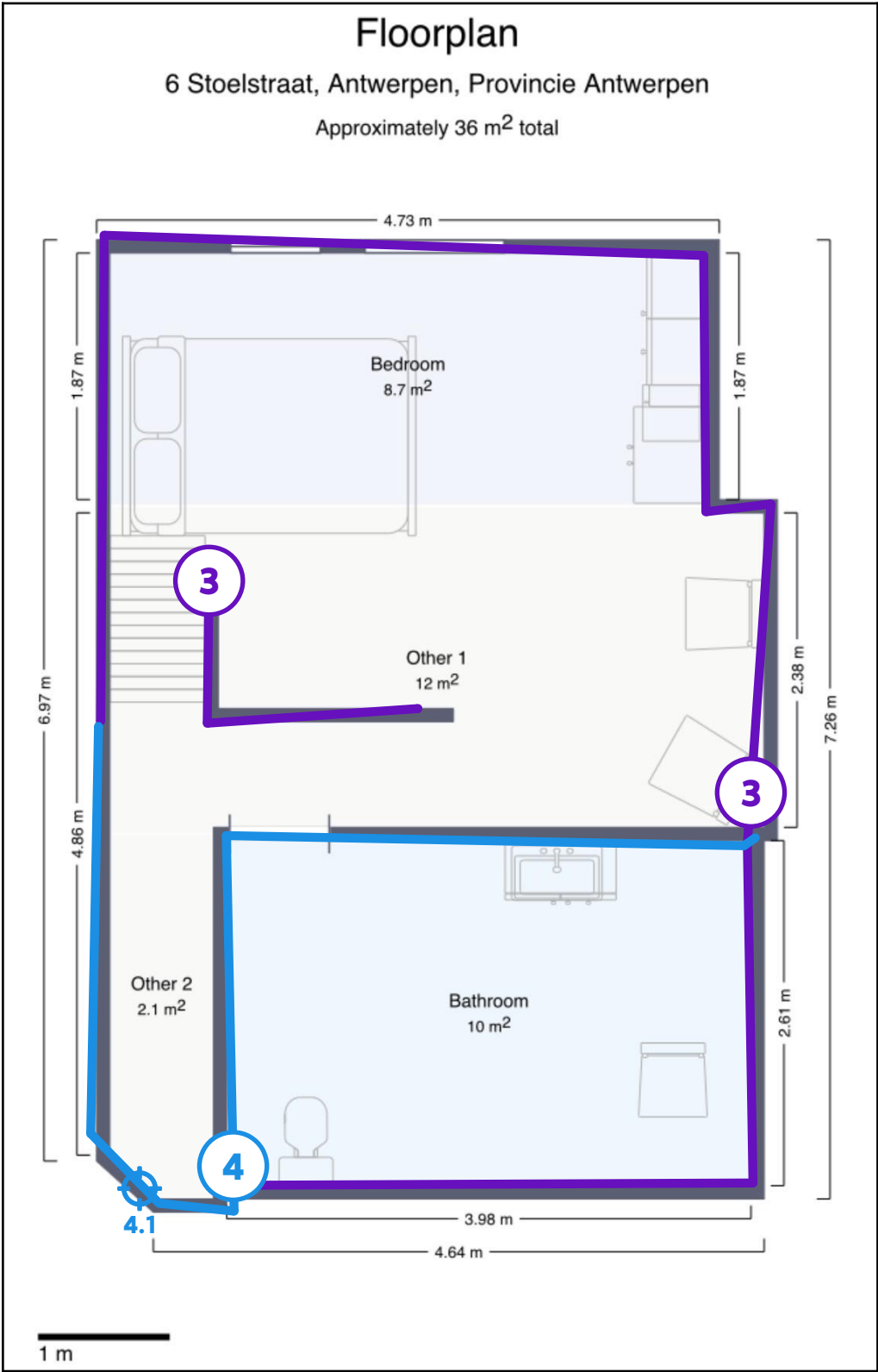
Legende van plan 1.10: 2de Verdieping
