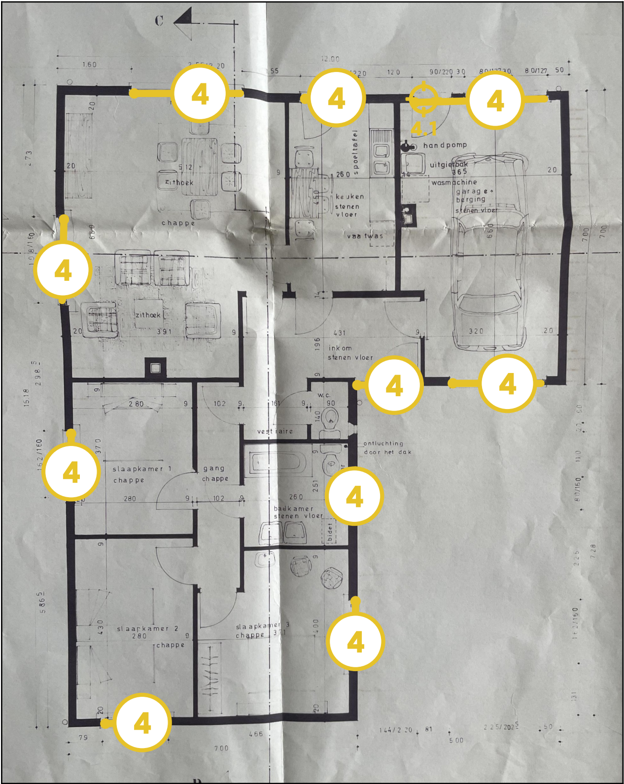
Legende van plan 1.6: Woning plan - Gelijkvloers
