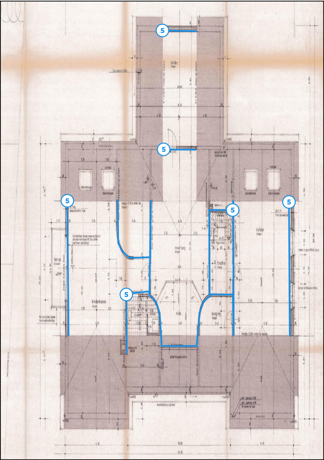
Legende van plan 1.6: plan verdieping - bezetting muren
