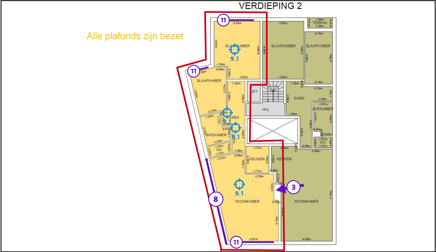
Legende van plan 1.2: Plan appartement
