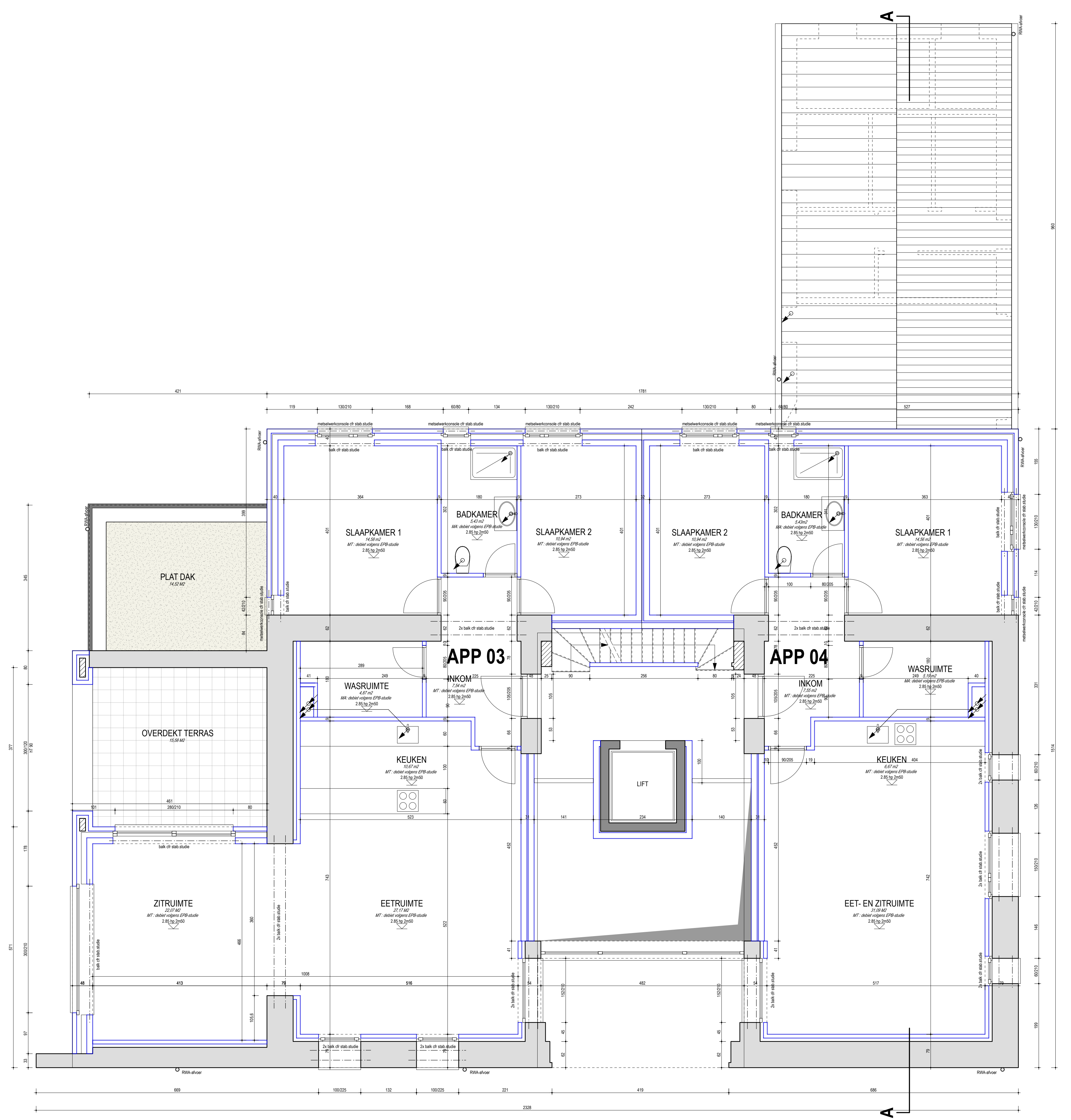
GRONDPLAN VERDIEPING 1 NIEUW schaal 1:50
