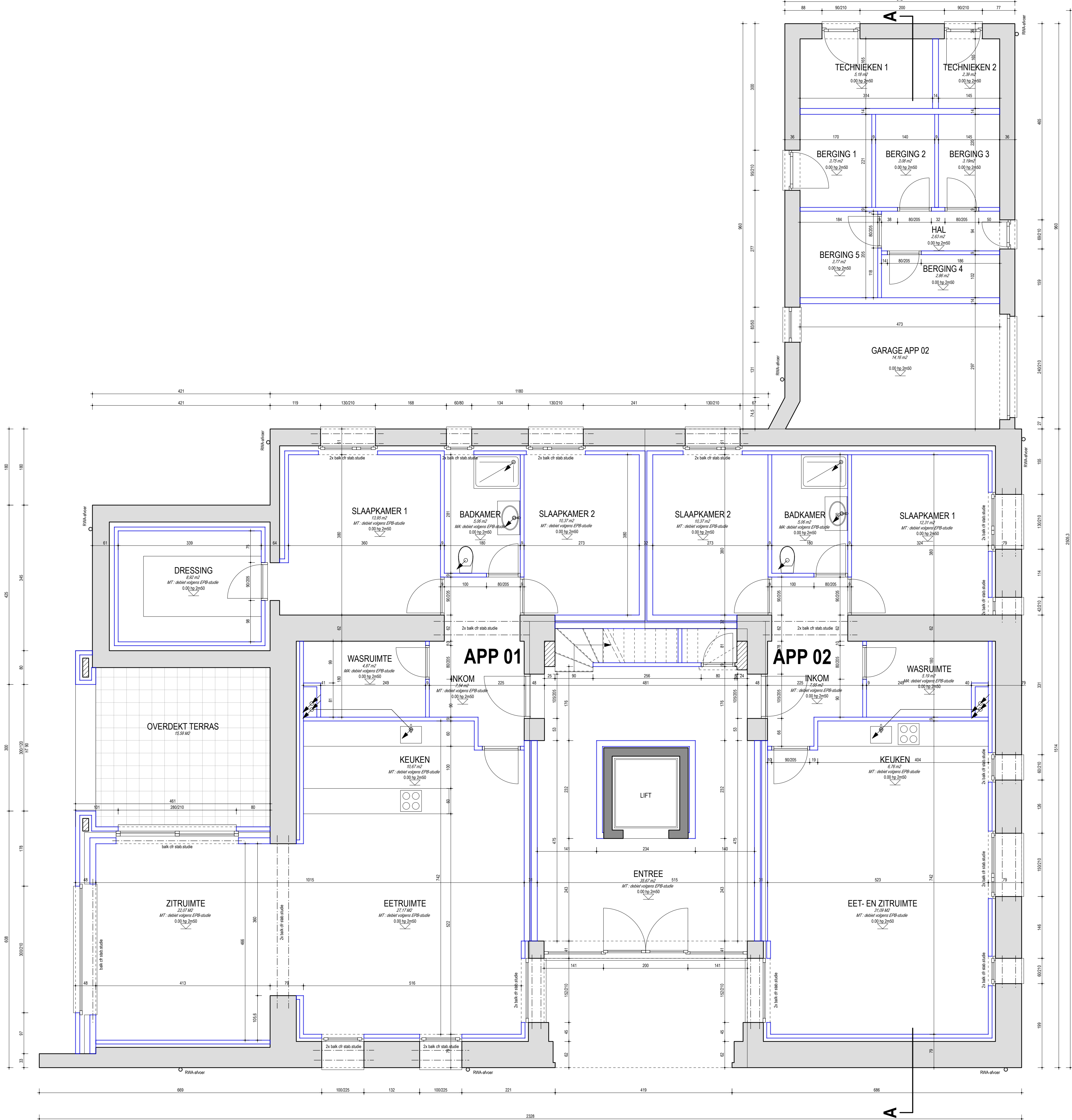
GRONDPLAN GELIJKVLOERS NIEUW schaal 1:50
