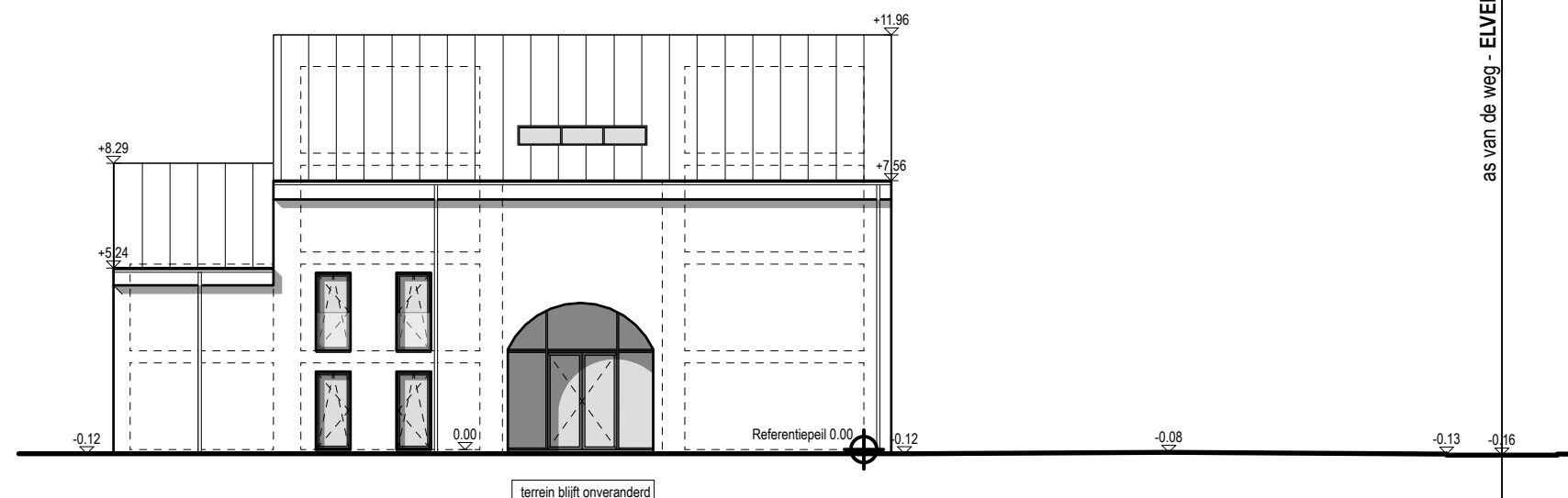
TERREINSNEDE BB NIEUW SCHAAL1/200
