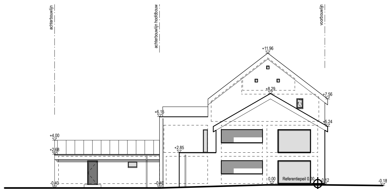
TERREINSNEDE AA NIEUW SCHAAL1/200
