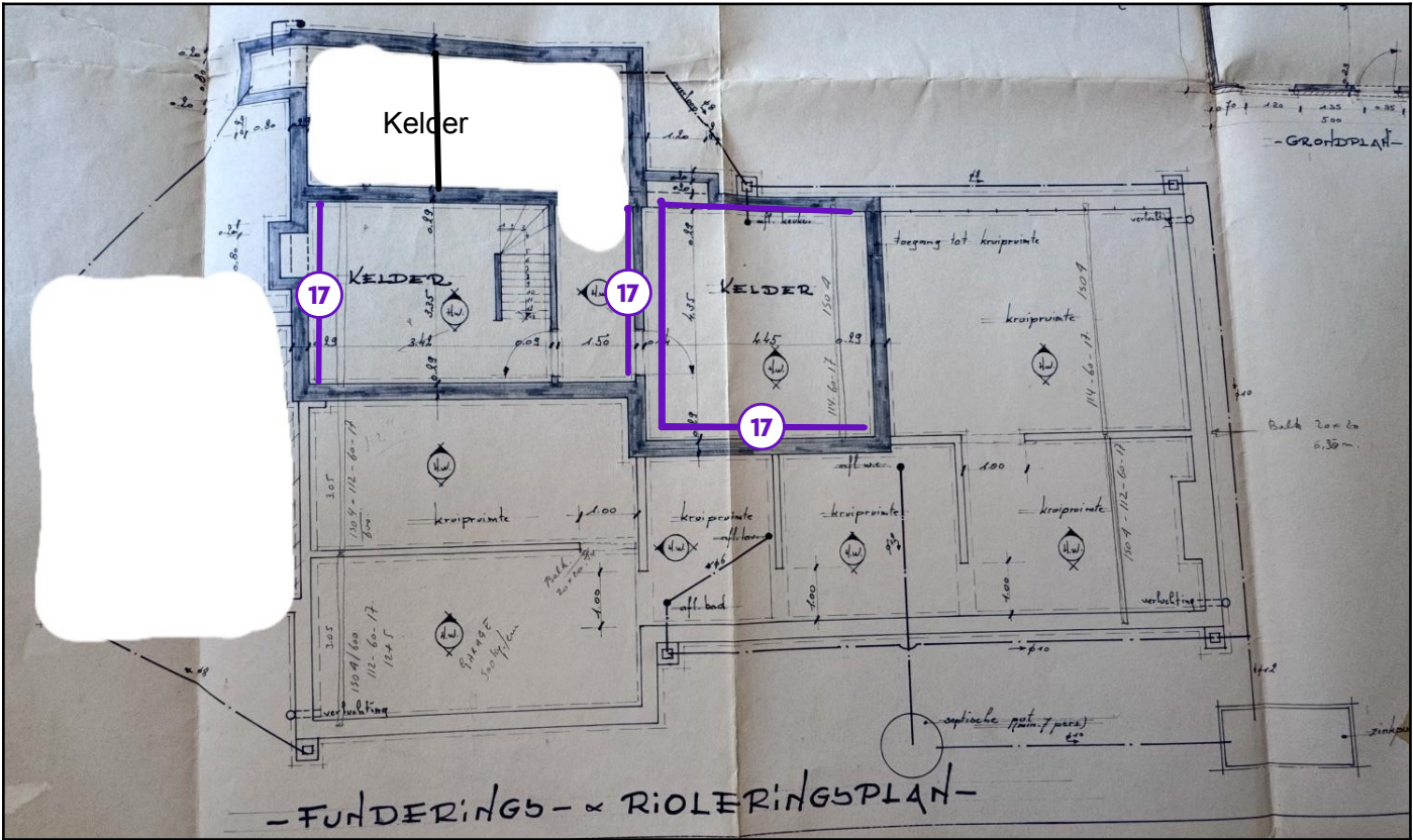
Legende van plan 1.2: Woning - kelder
