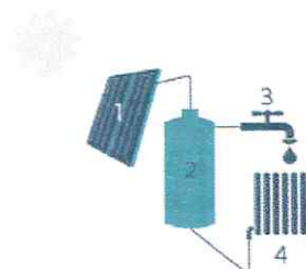
1. Zonnecollector | 2. Opslagvat zonneboiler | 3. Sanitair warm water | 4. Afgiftelement voor ruimteverwarming (optioneel)
