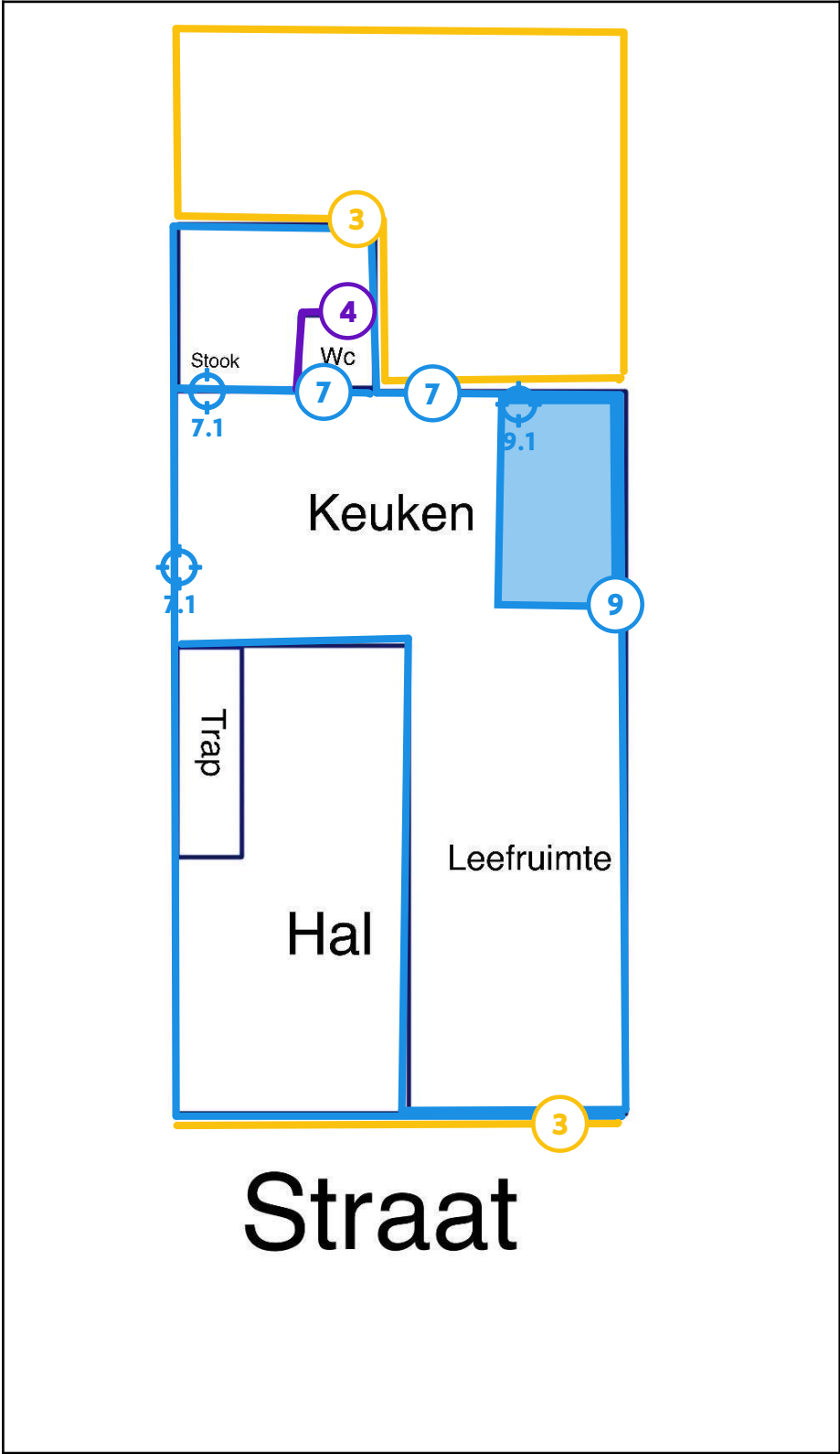
Legende van plan 1.8: Gelijkvloers
