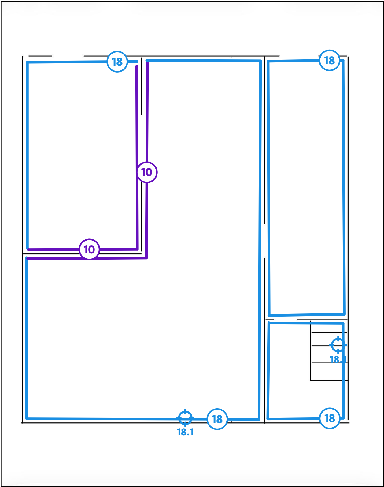
Legende van plan 1.3: Gelijkvloers voorbouw
