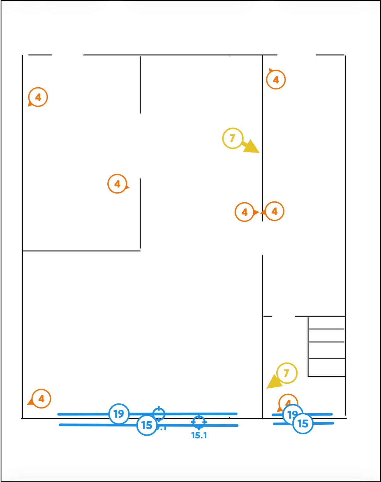
Legende van plan 1.5: Gelijkvloers voorbouw
