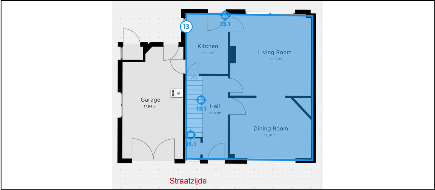
Legende van plan 1.6: Gelijkvloers
