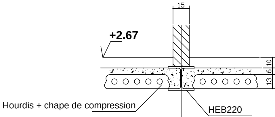
COUPE 3-3
