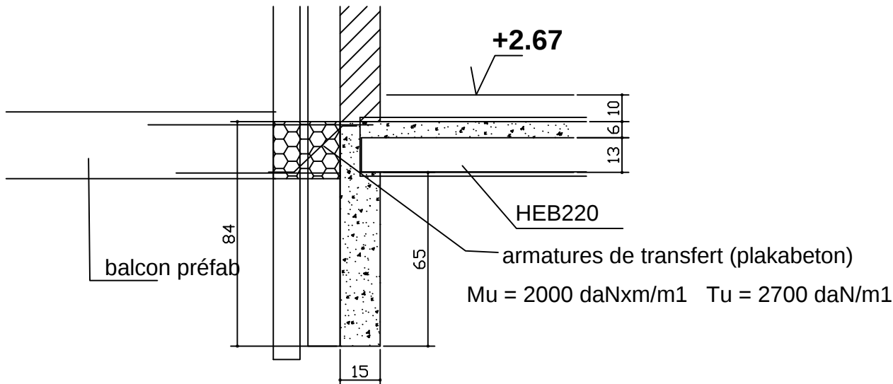
COUPE 6-6
