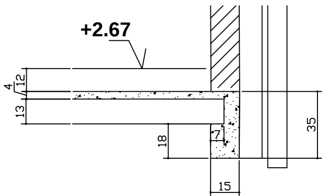
COUPE 4-4
