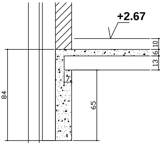
COUPE 5-5
