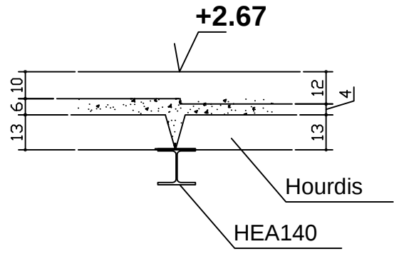
COUPE 1-1
