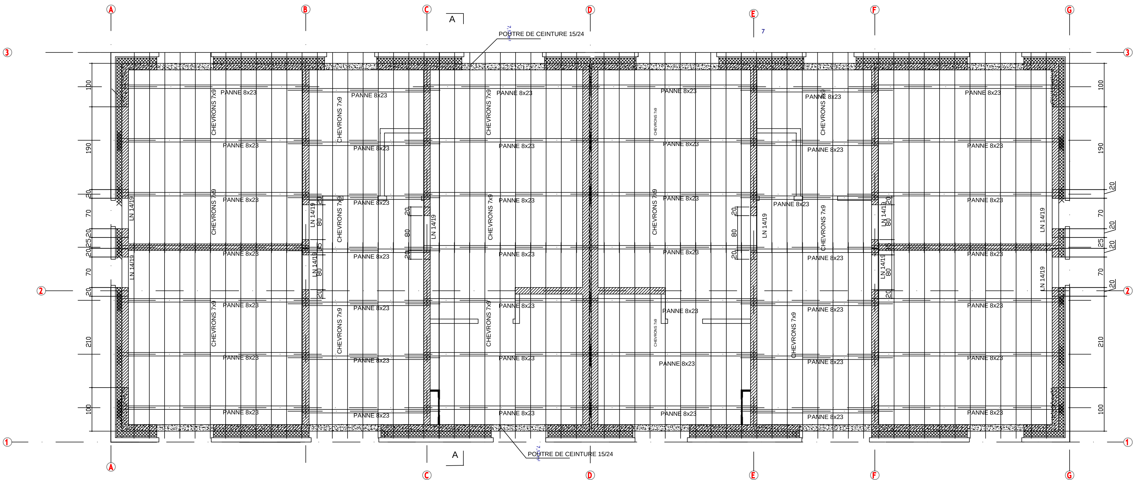
VUE EN PLAN TOITURE
