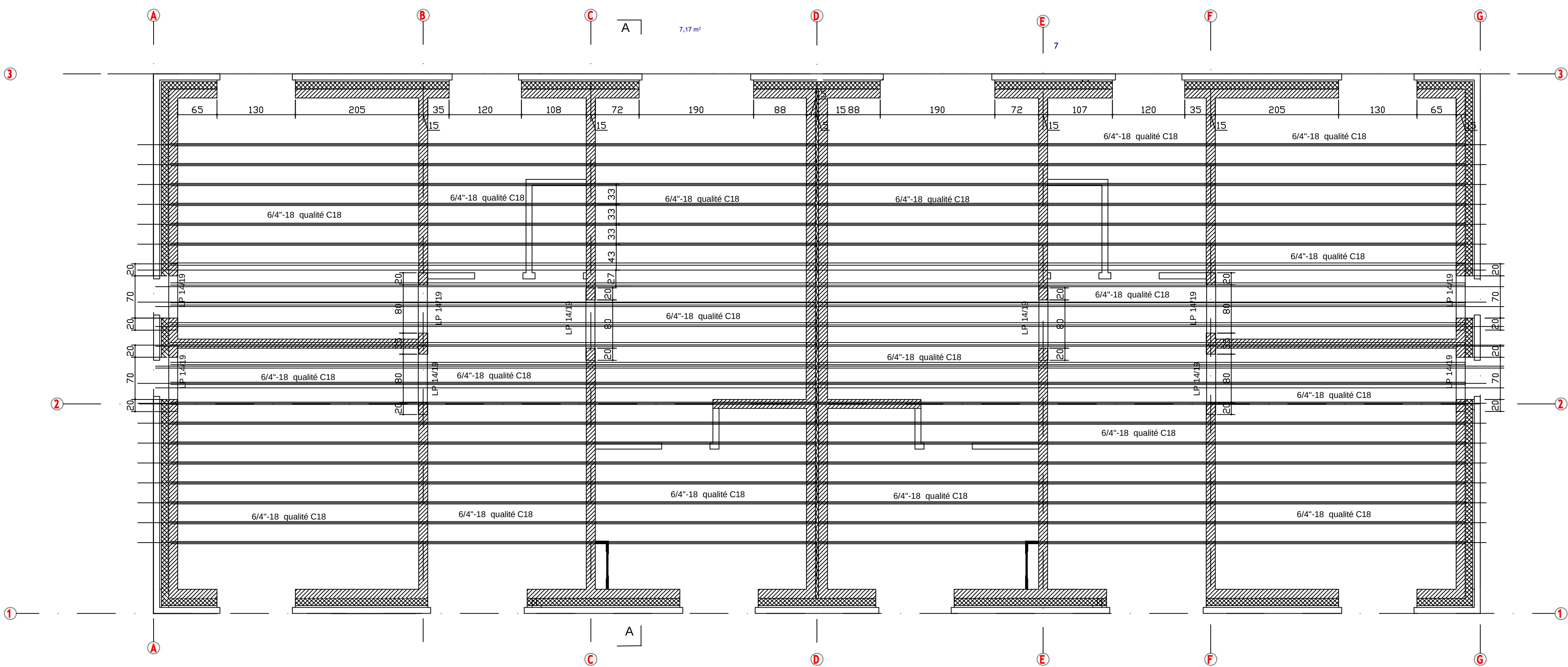
VUE EN PLAN PLANCHER COMBLES
