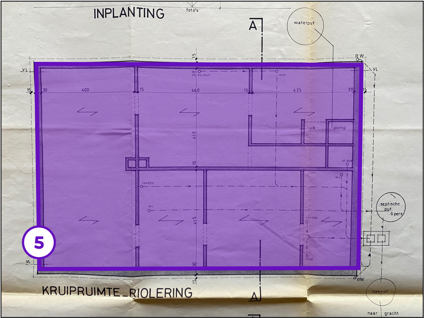
Legende van plan 1.3: Kruipkelder plan
