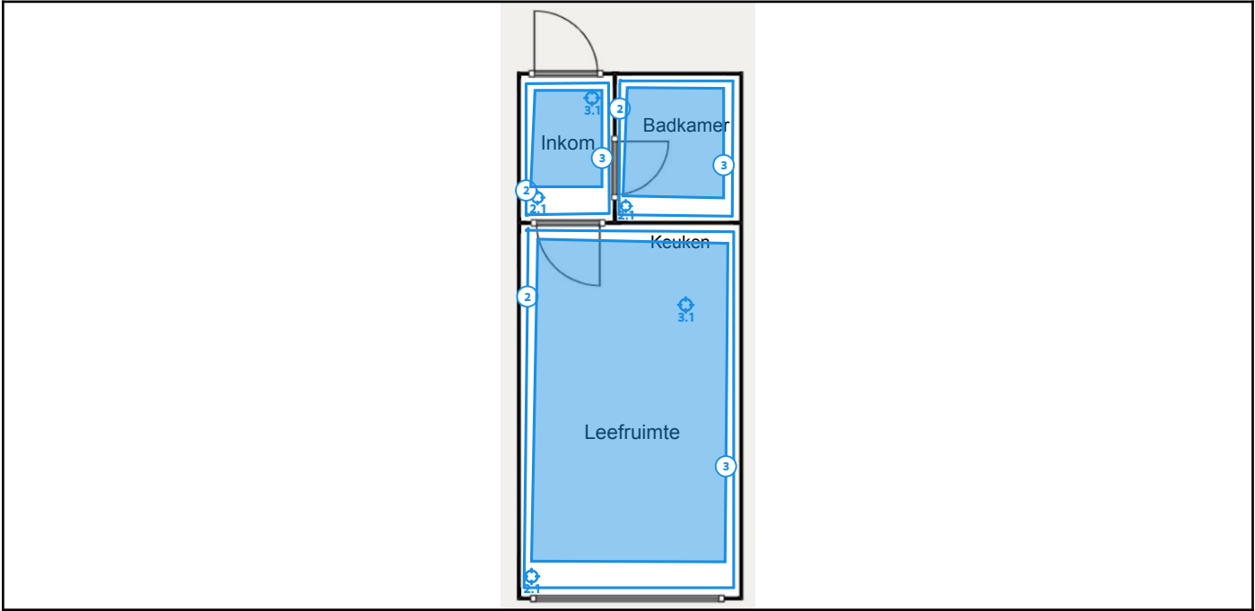
Legende van plan 1.2: Grondplan appartement 0411
