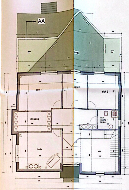
VERDIEPING 1 1/100
