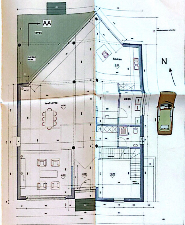
GELIJKVLOERS 1/100
