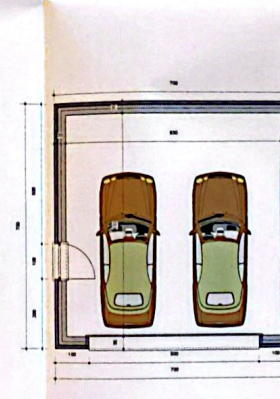
GELIJKVLOERS 1/100
