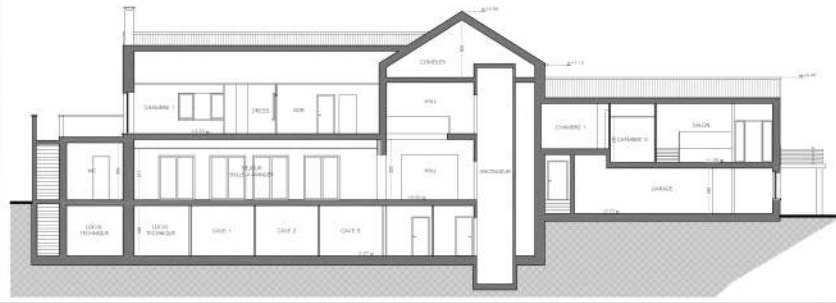
Coupe A
