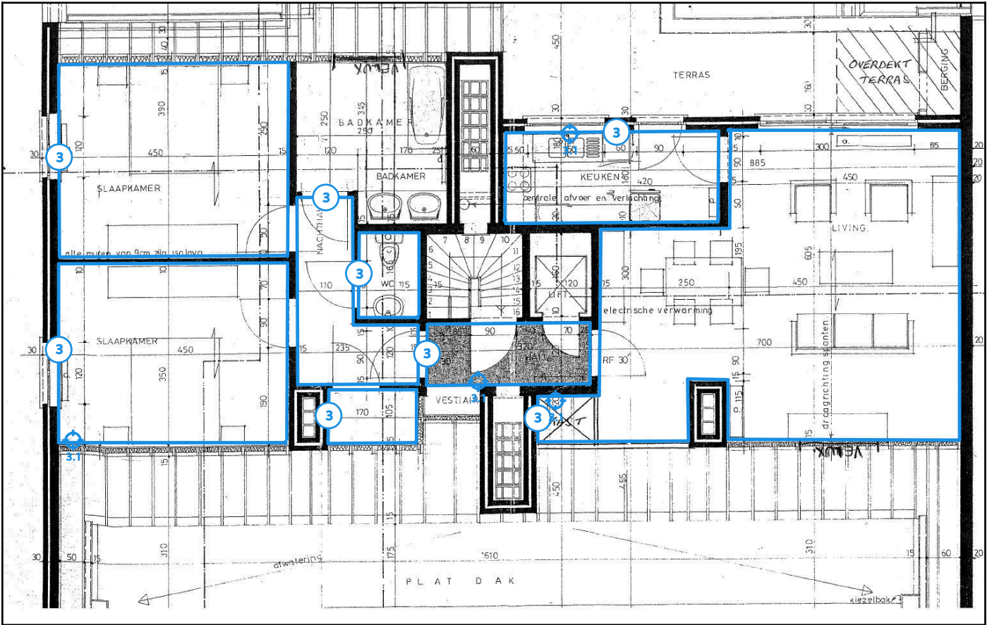
Legende van plan 1.1: Grondplan
