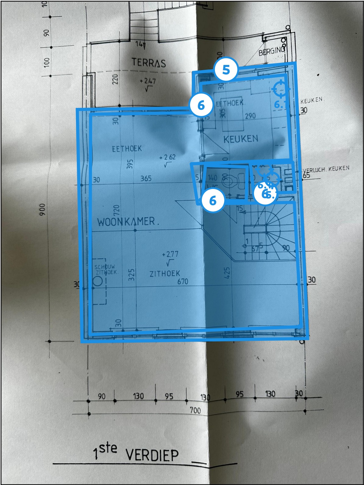
Legende van plan 1.4: Grondplan eerste verdiep wanden en plafonds
