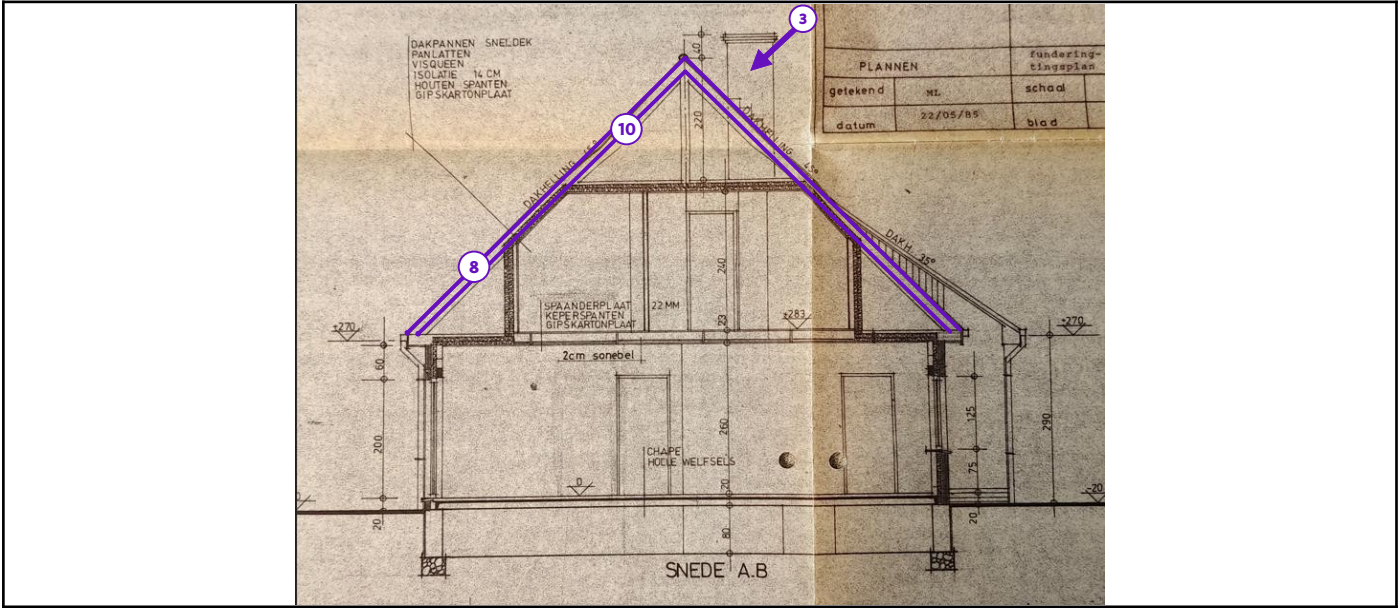
Legende van plan 1.4: Doorsnede
