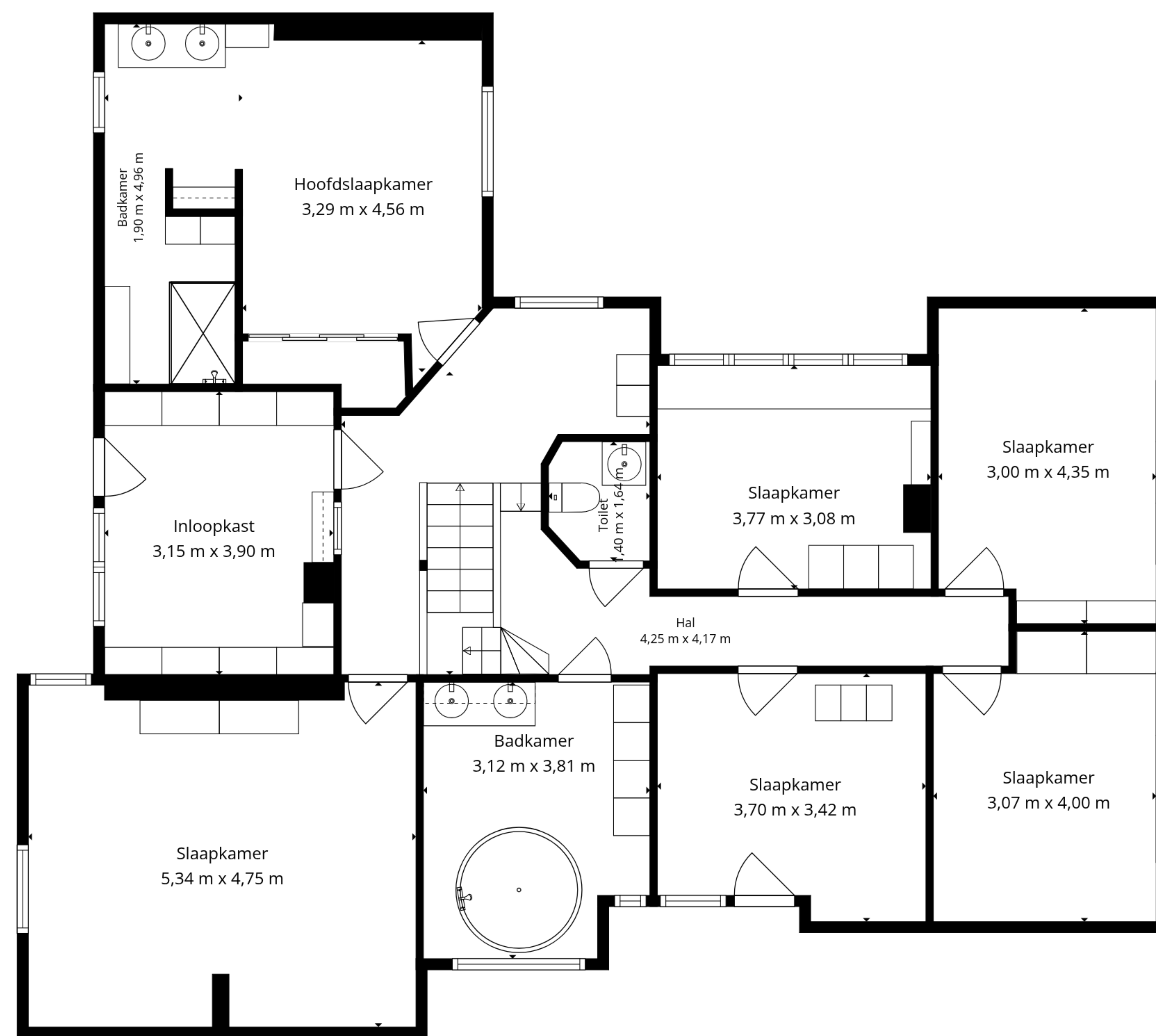
2e Verdieping
