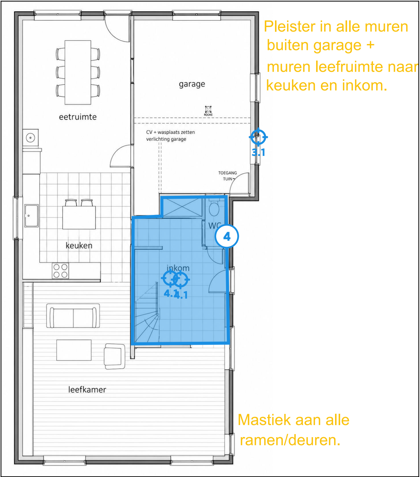
Legende van plan 1.1: Hoofdgebouw gelijkvloers
