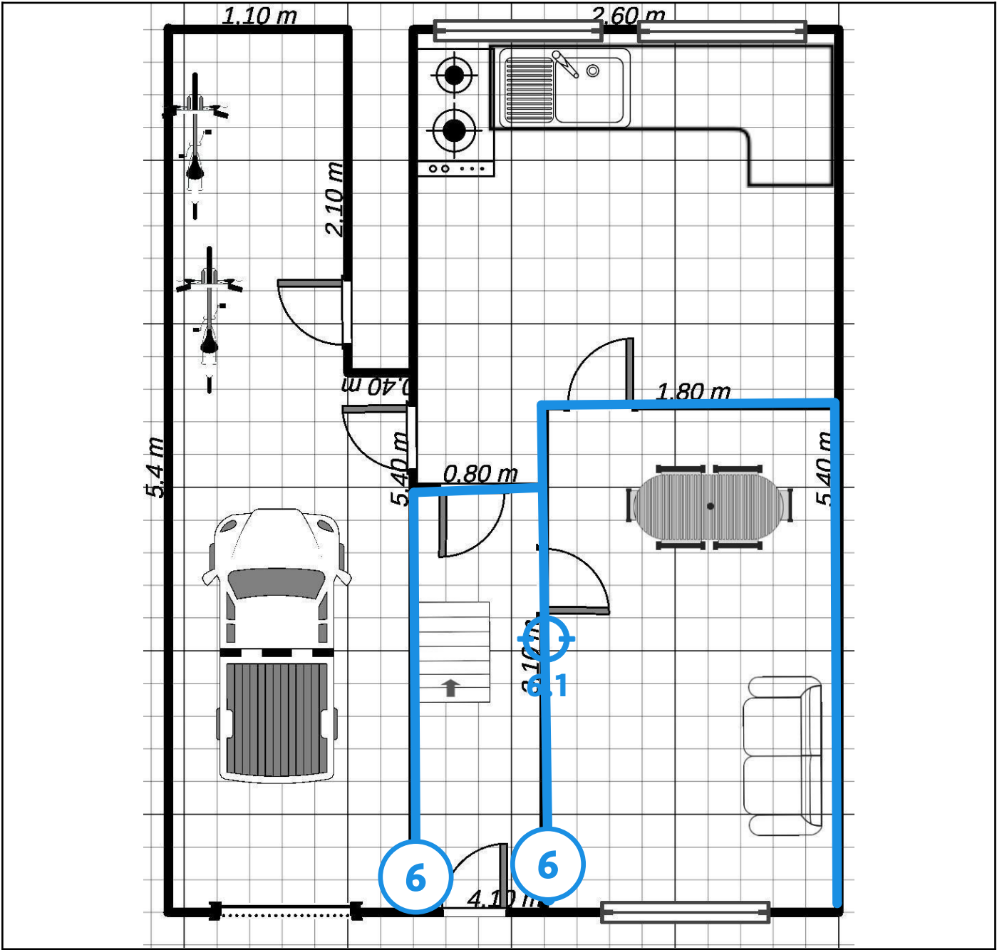
Legende van plan 1.4: Gelijkvloers 1.2
