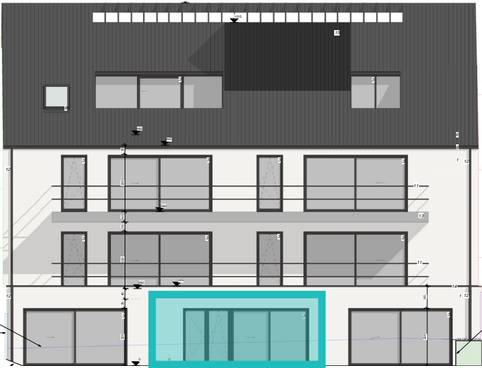
Achtergevel
