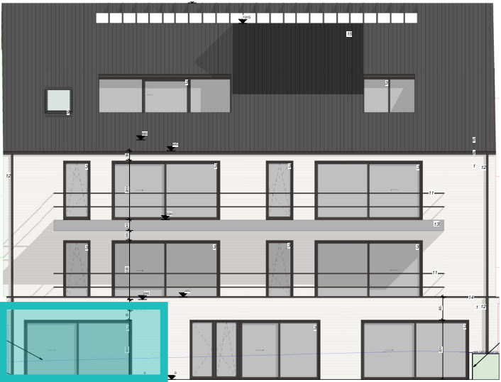
Achtergevel
