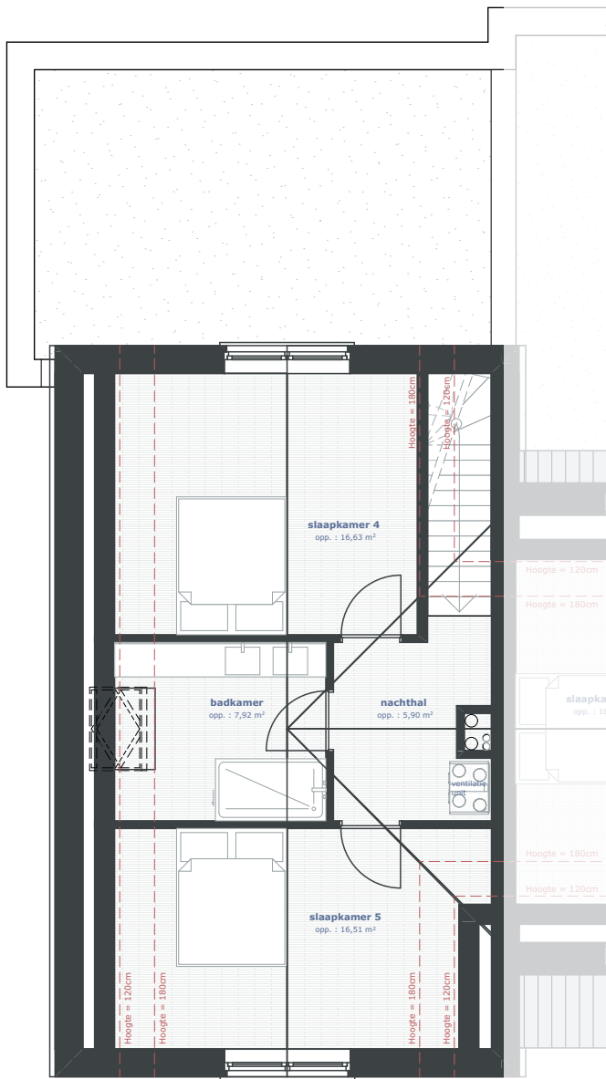
NIVO +2 - 1:100
