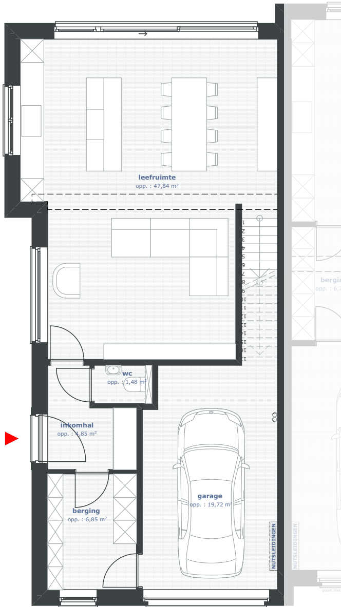
NIVO +0 - 1:100
