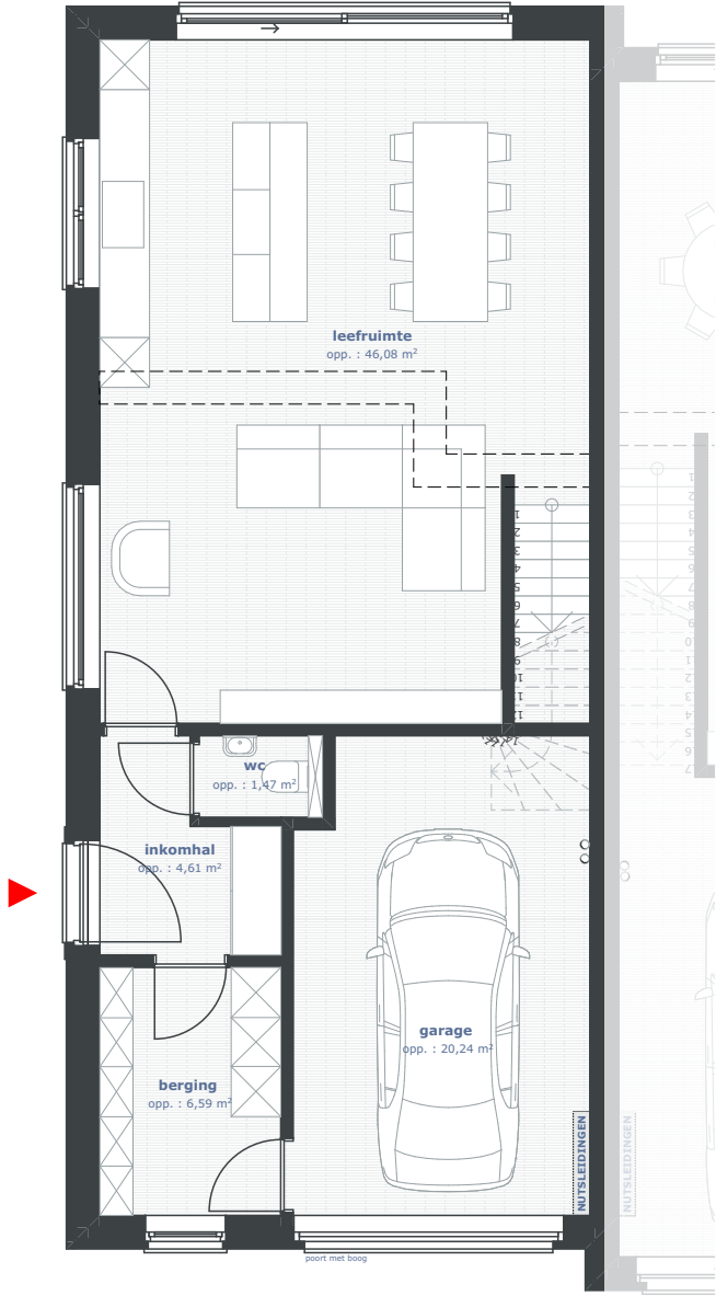
NIVO +0 - 1:100
