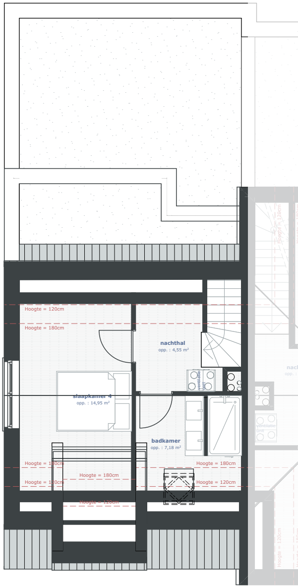
NIVO +2 - 1:100
