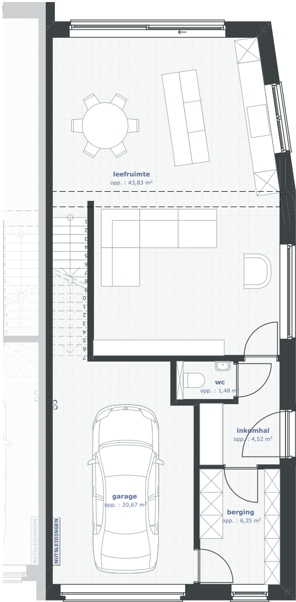
NIVO +0 - 1:100
