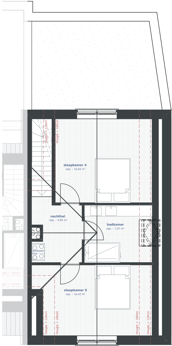
NIVO +2 - 1:100
