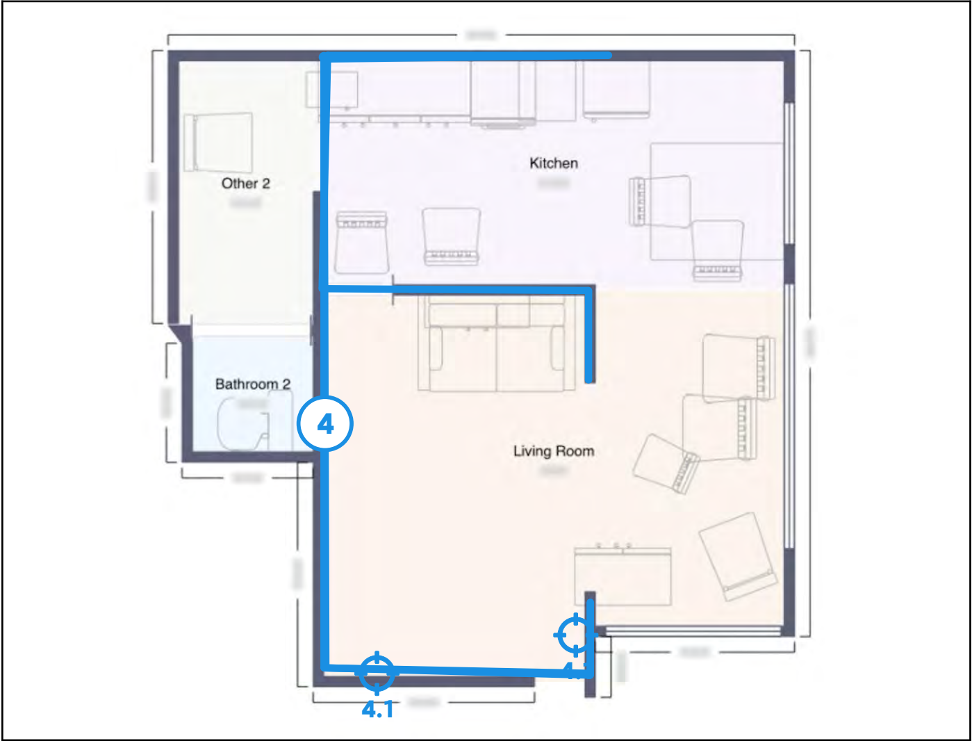
Legende van plan 3.1: Gelijkvloers
