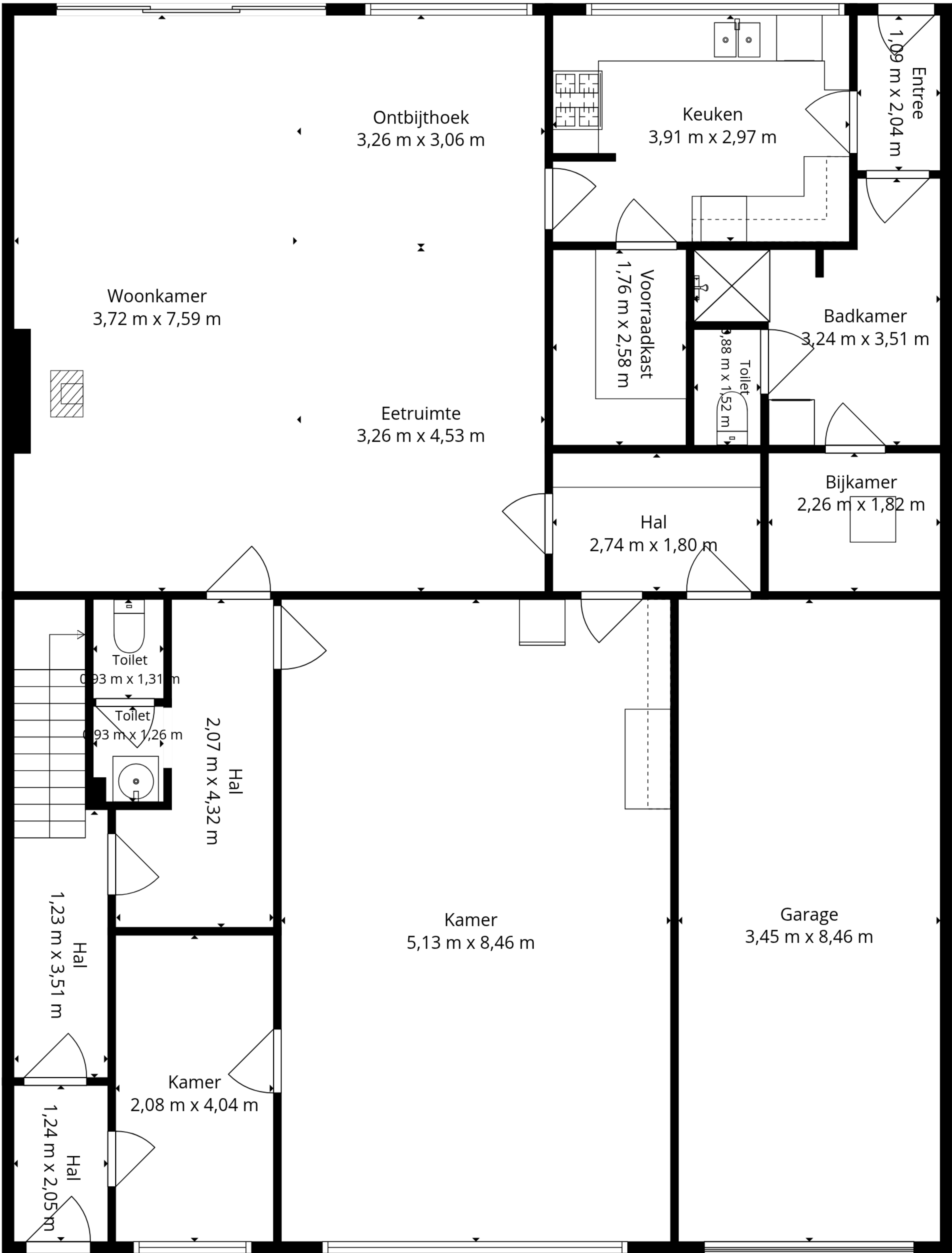
1e Verdieping
