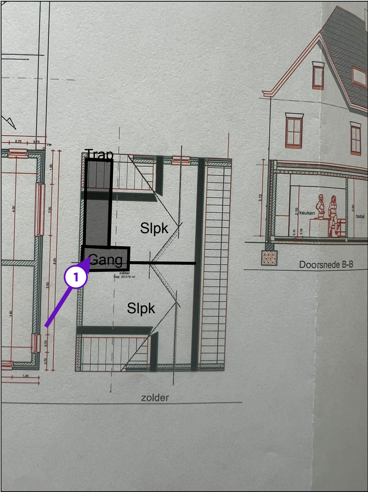
Legende van plan 1.6: zolder schouw
