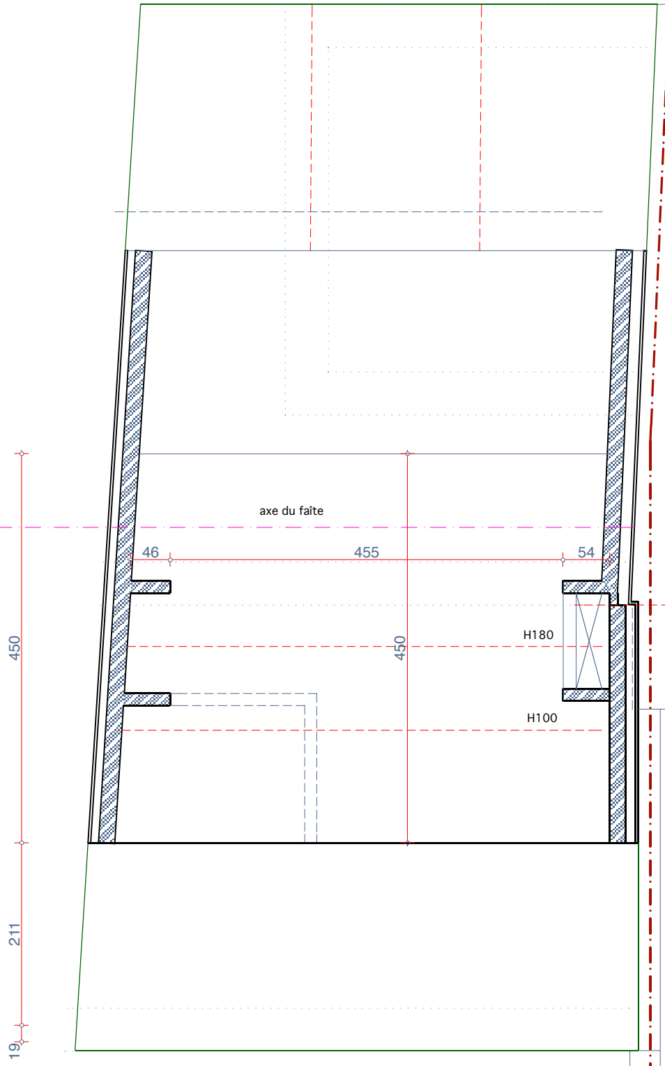
PLAN du 4 ° étage
