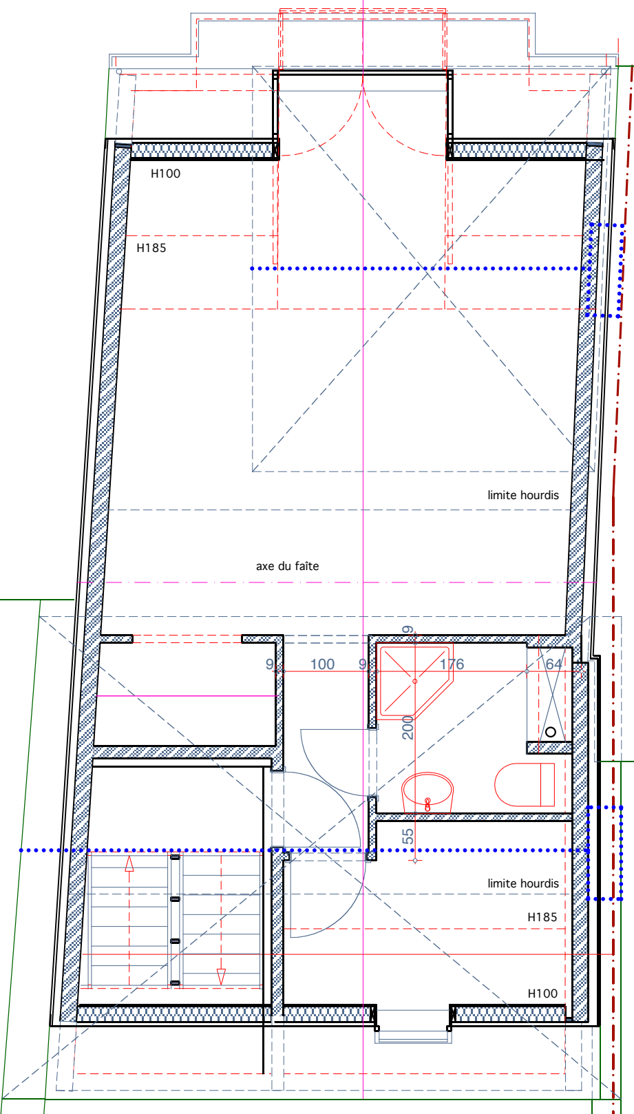
PLAN du 3 ° étage
